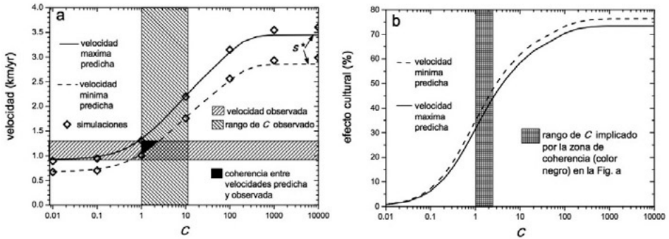
Fig. 4 – Velocidades predichas por un modelo de la propagación del frente neolítico en Europa en función de la intensidad de transmisión cultural C (a). Estas velocidades implican que el porcentaje de la difusión cultural fue entre un 32% y un 48% (b), según lo cual la difusión démica (movimiento de poblaciones) fue más importante que la difusión cultural (movimiento de ideas) a escala continental (adoptado de FORTE 2012).
