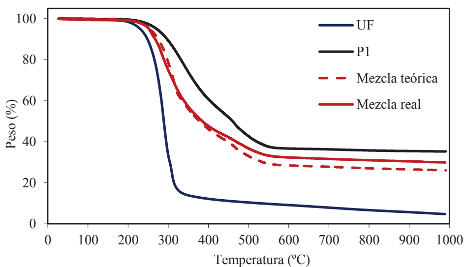
Figura 7.12. Curvas TG de la breya P1, la resina UF y sus mezclas teórica y real.
