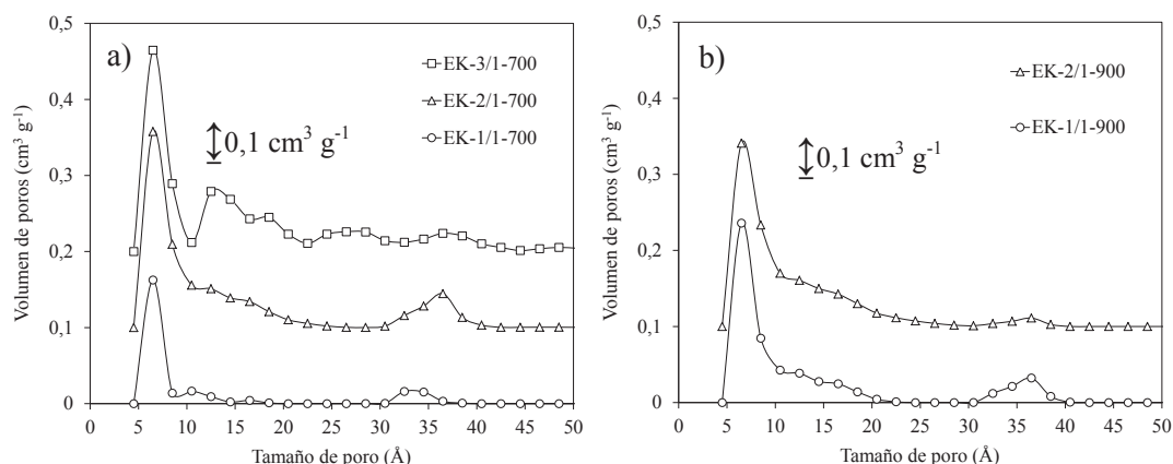
Figura 5.12. Distribuciones de tamaño de poros (QSDFT) para las fibras estabilizadas no carbonizadas activadas con KOH a 700 (a) y 900 °C (b).
