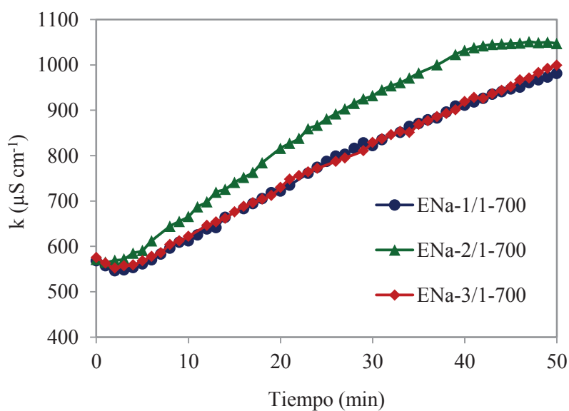
Figura 9.4. Curvas de conductividad iónica frente al tiempo para las fibras estabilizadas activadas con NaOH.
