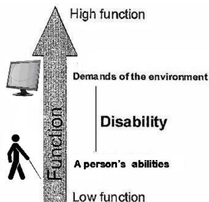
El esquema del gap. Adaptado de Aslaksen et al. (1997)
