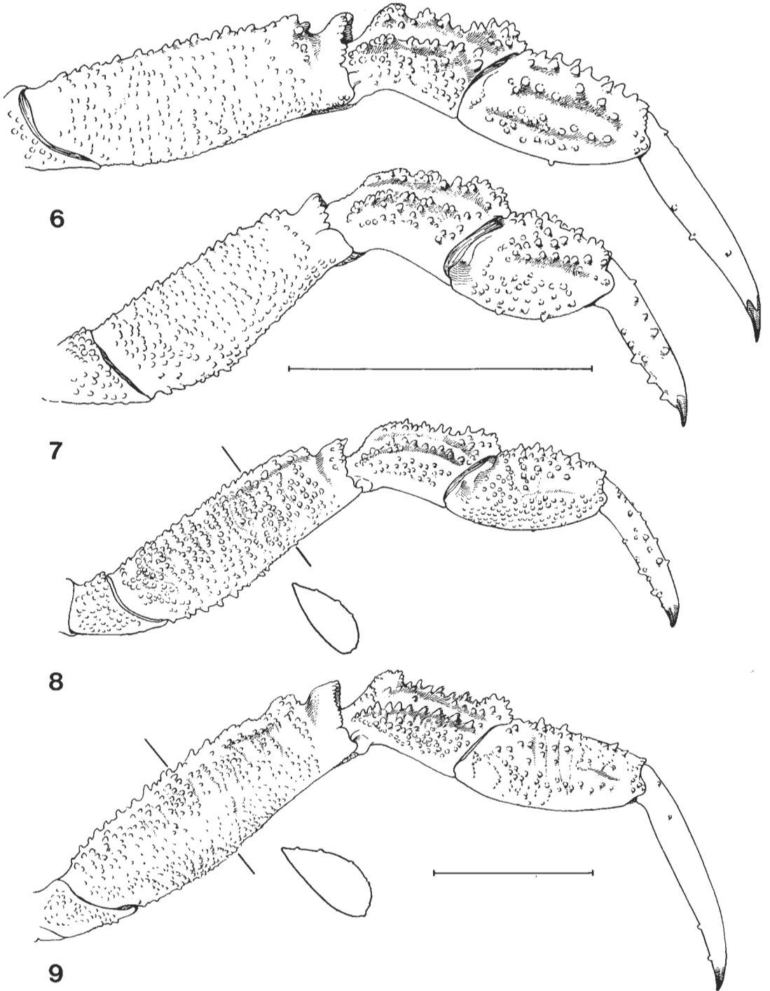
FIG. 6-9. — Pattes ambulatoires : 6, 7, Monodaeus arnaudi sp. nov., holotype, ♂ 10,4 × 15,1 mm, Nouvelle-Amsterdam (MP-B9582) : 6, P4 ; 7, P5. — 8, 9, M. cristulatus sp. nov., holotype, ♂ 16,4 × 23,9 mm, Namibie (MP-B17498) : 8, P4 ; 9, P5 ; au-dessous, une coupe transversale du mérus qui montre la crête du bord supérieur. (Échelles = 0,5 cm.)
