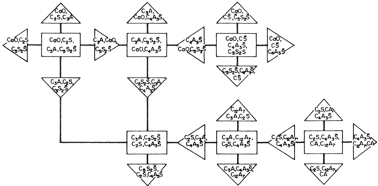
Fig. 7.- Diagrama esquemático de la relación de fases condensadas en la zona rica en cal del sistema \text{CaO-Al}_2\text{O}_3\text{-SiO}_2\text{-SO}_3 a \sim 1.000^\circ\text{C} (27).
