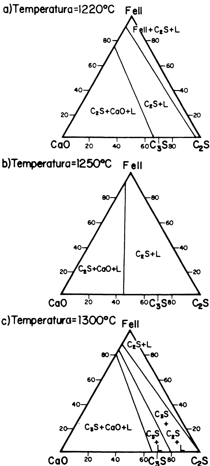
Fig. 3.- Secciones isotérmicas en el sistema CaO-C 2 S-Fell a) 1.220°C, b) 1.250°C y c) 1.300°C (40). Fig. 3.- Isothermal sections of the CaO-C 2 S-Fell system at: a) 1.220°C, b) 1.250°C y c) 1.300°C (40).
