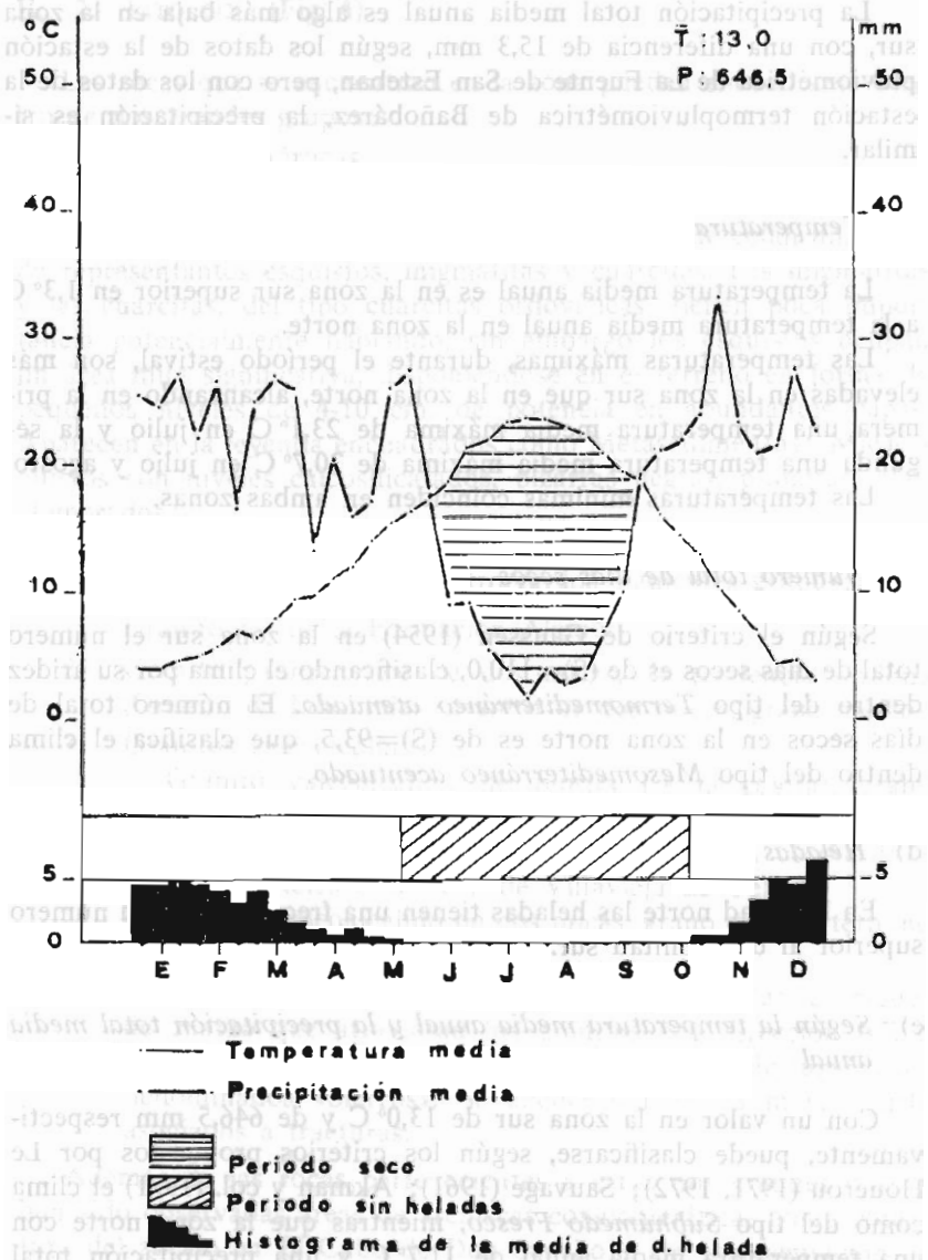
Fig. 3.- DIAGRAMA CLIMÁTICO (1958-1972)
