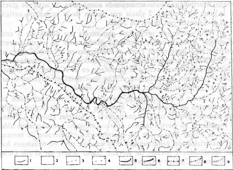
FIG. 6.— CUENCAS HIDROGRAFICAS
