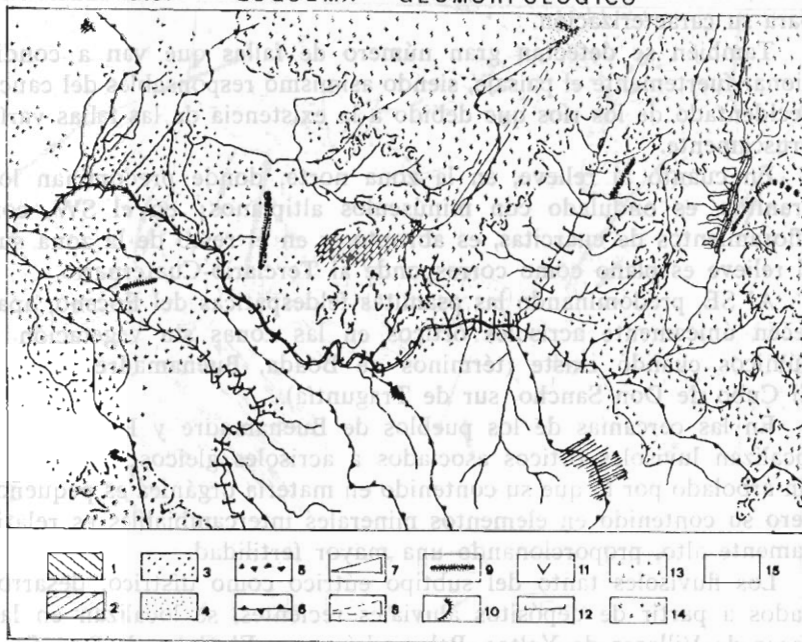
FIG. 5.— ESQUEMA GEOMORFOLOGICO
