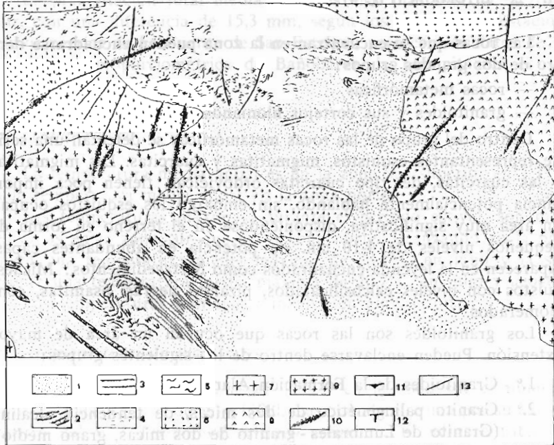
FIG. 4.— ESQUEMA LITOLÓGICO
