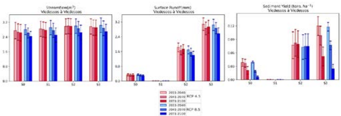
Figure 8.10. Débit annuel moyen ( m^3.s^{-1} ), ruissellement de surface ( Hm^3 ) et l'apport en sédiments ( tons.ha^{-1} ) à Vicdessos pour chaque période et chaque scénario d'émission selon quatre scénarios de gestion. (S0: base; S1: pâturages transformés en forêt; S2: 30% de la superficie forestière totale est coupée à blanc; S3: pâturages transformés en forêt et 30% de la superficie forestière totale est coupée à blanc).
