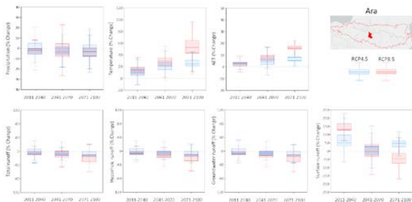
Figure 6.5. Variation par rapport à la période de contrôle (1961-2005) des précipitations, de la température, de l'évapotranspiration et des débits de décharge totale, de flux hyporréique et souterrain, ainsi que du ruissellement superficiel, en faisant la moyenne des valeurs de chacune de ces variables pour les périodes 2011-2040, 2041-2070 et 2071-2100.
