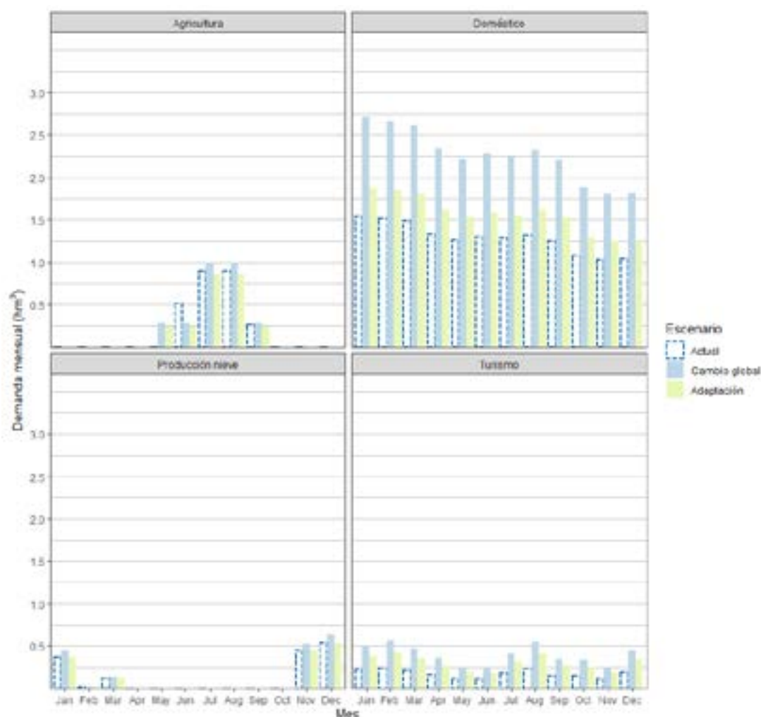
Figure 3.9. Demanda mensual d'eau (hm 3 ) pour des usages domestique, touristique, de production de neige et agricole dans les scénarios considérés pour 2050.
