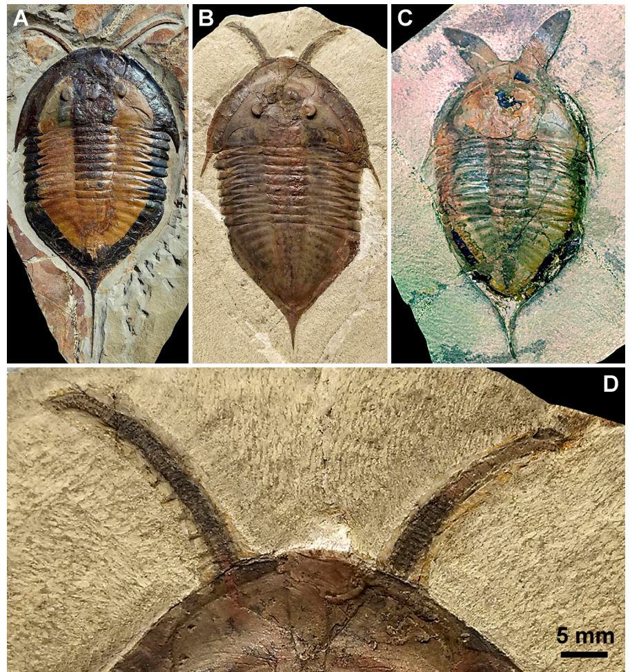
Fig. 2.- Megistaspis (Ekeraspis) hammondi Corbacho y Vela. Biota de Fezouata, Tremadociense superior del norte de Zagora (Marruecos). Ejemplares observados a la venta en circuitos comerciales y sitios de internet. A, ejemplar con caparazón bien conservado, y con la doblez ventral contorneada en negro por su posible concentración en materia orgánica; las antenas son largas y estrechas, la de la derecha tiene más de 45 podómeros desiguales y sus bordes laterales están tallados en la roca. B, ejemplar con puntas genales y pigidio esculpido en su parte posterior; las antenas son notablemente más gruesas, con 30-35 podómeros rectangulares, algunos con espinas abaxiales (detalle en D). C, ejemplar con la antena izquierda (línea clara) conservada en el seno de una "oreja de gato" como las que algunos preparadores tallan en esta especie.
