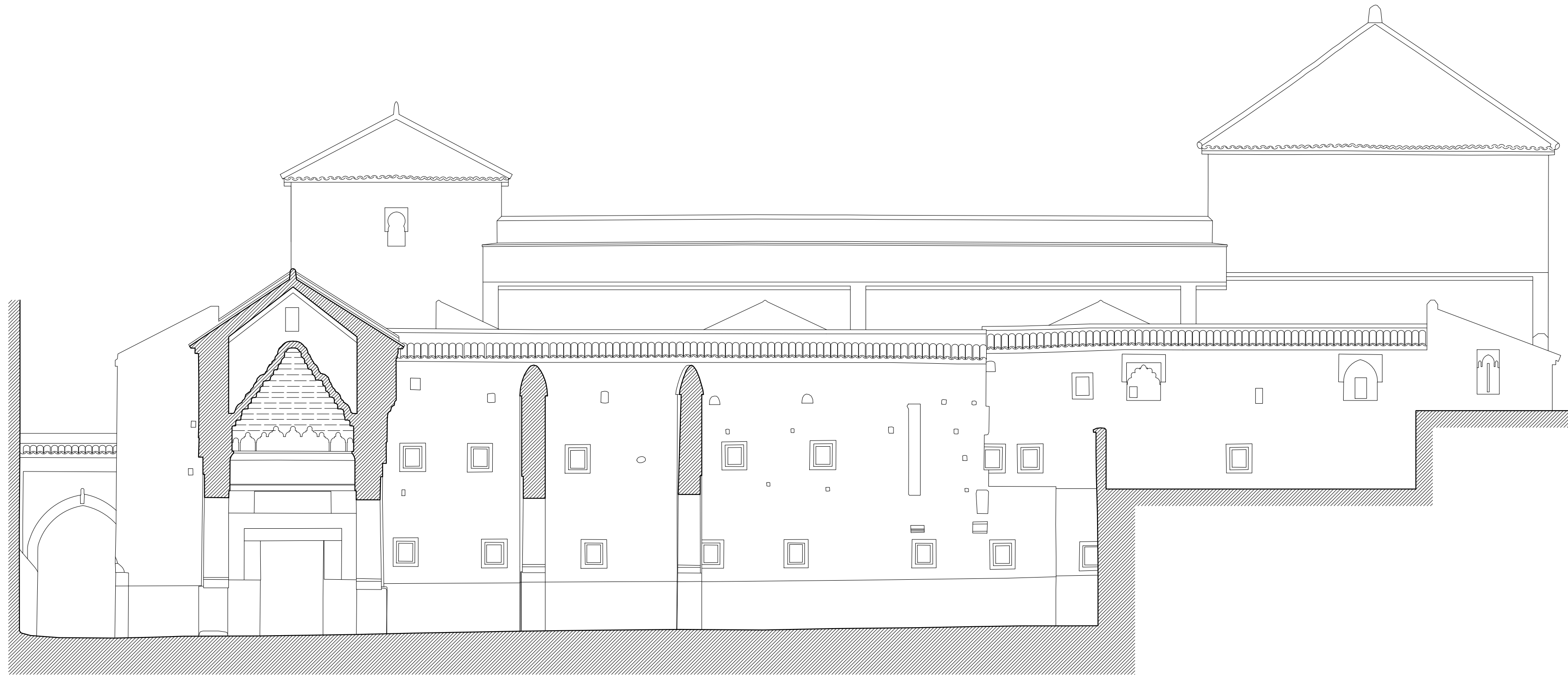
FACHADA OESTE
