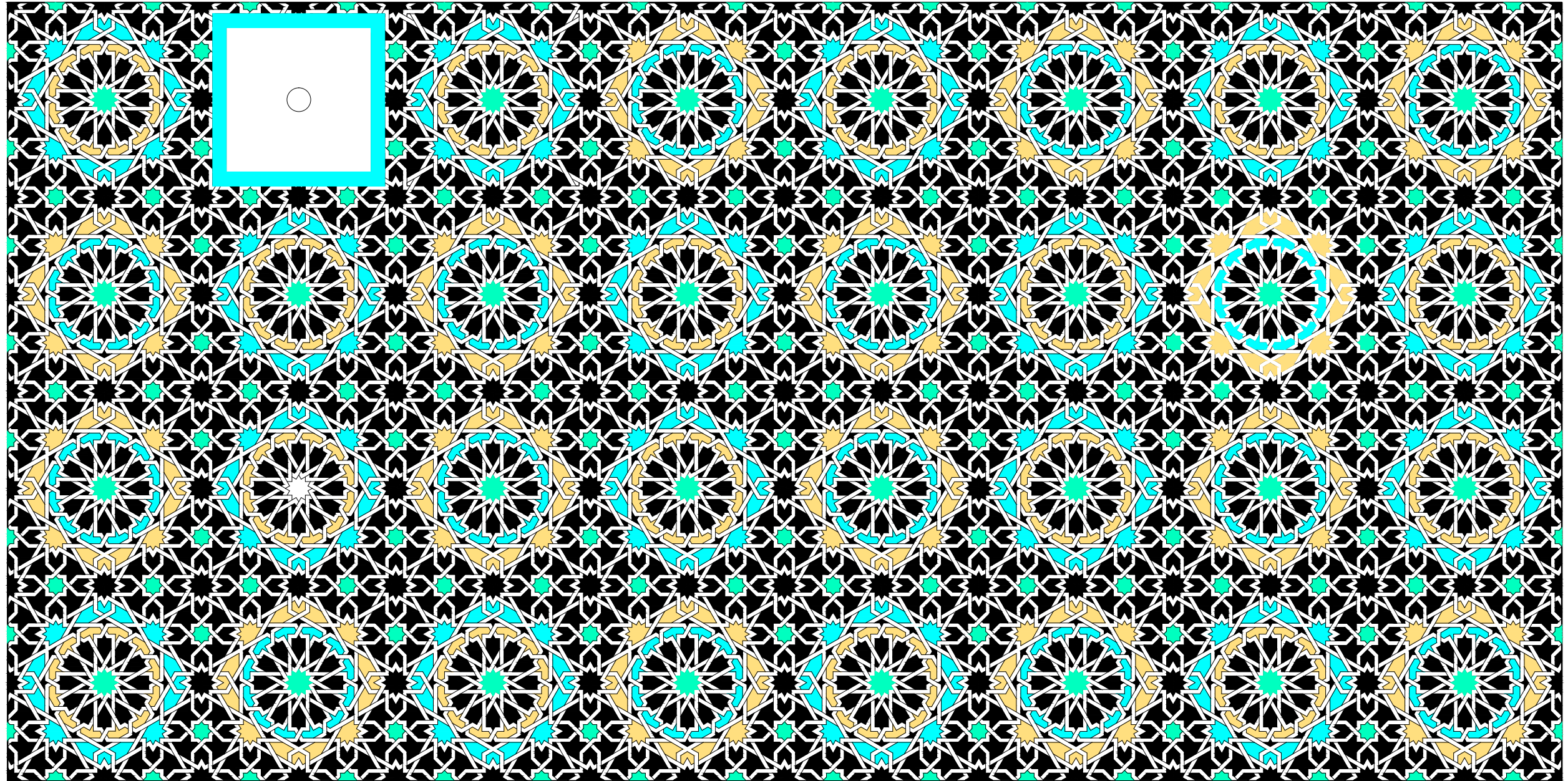
0 1 m ALICATADO DE LA ALBERCA DE LA QUBBA AL-JAMSIYYA DEL PALACIO AL-BADI' DE MARRAKECH ESCUELA DE ESTUDIOS ÁRABES, CSIC. A. ALMAGRO / Arq. Julio 2016
