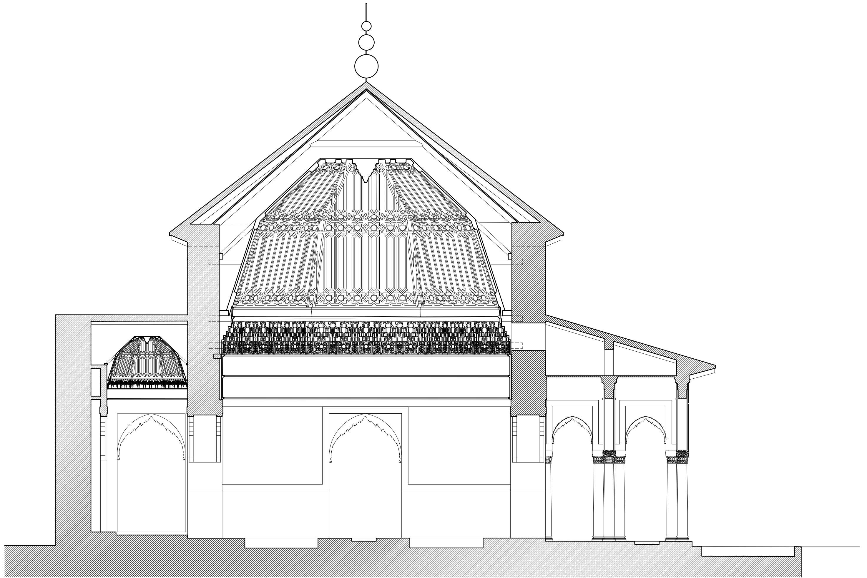
PALACIO AL-BADI'. MARRAKECH. PABELLÓN OESTE. SECCIÓN O-E. HIPÓTESIS ANTONIO ALMAGRO / arquitecto ESCUELA DE ESTUDIOS ÁRABES, CSIC
