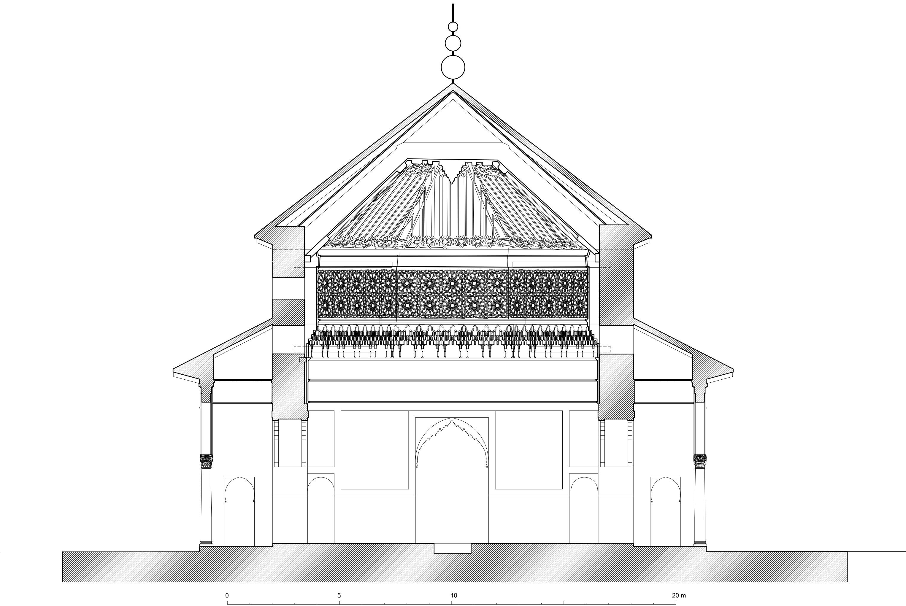
PALACIO AL-BADI'. MARRAKECH. PABELLÓN OESTE. SECCIÓN N-S HIPÓTESIS ANTONIO ALMAGRO / arquitecto ESCUELA DE ESTUDIOS ÁRABES, CSIC
