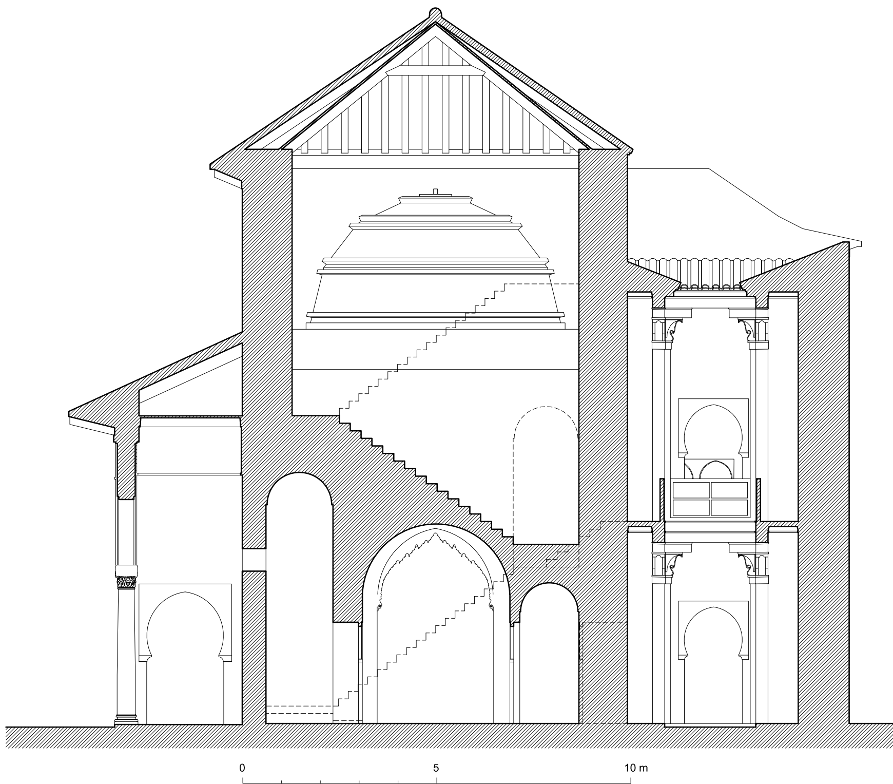
PALACIO AL-BADI' DE MARRAKECH. SALÓN NORTE. SECCION POR ESCALERA. HIPÓTESIS A. ALMAGRO (arq. Escuela de Estudios Árabes, CSIC) 2008-2016
