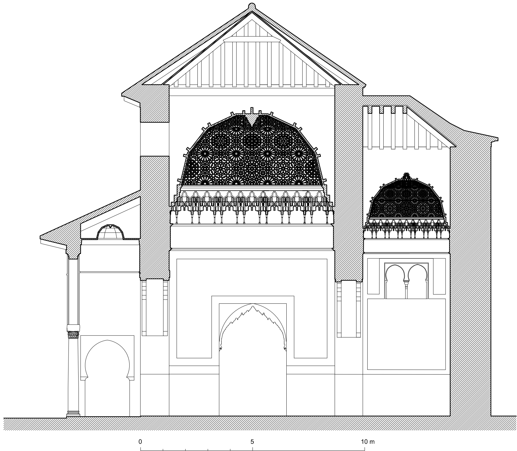
PALACIO AL-BADI DE MARRAKECH. SALÓN NORTE. SECCION LONGITUDINAL. HIPÓTESIS A. ALMAGRO Ibarra, Escuela de Estudios Árabes, CSIC 2005-2016
