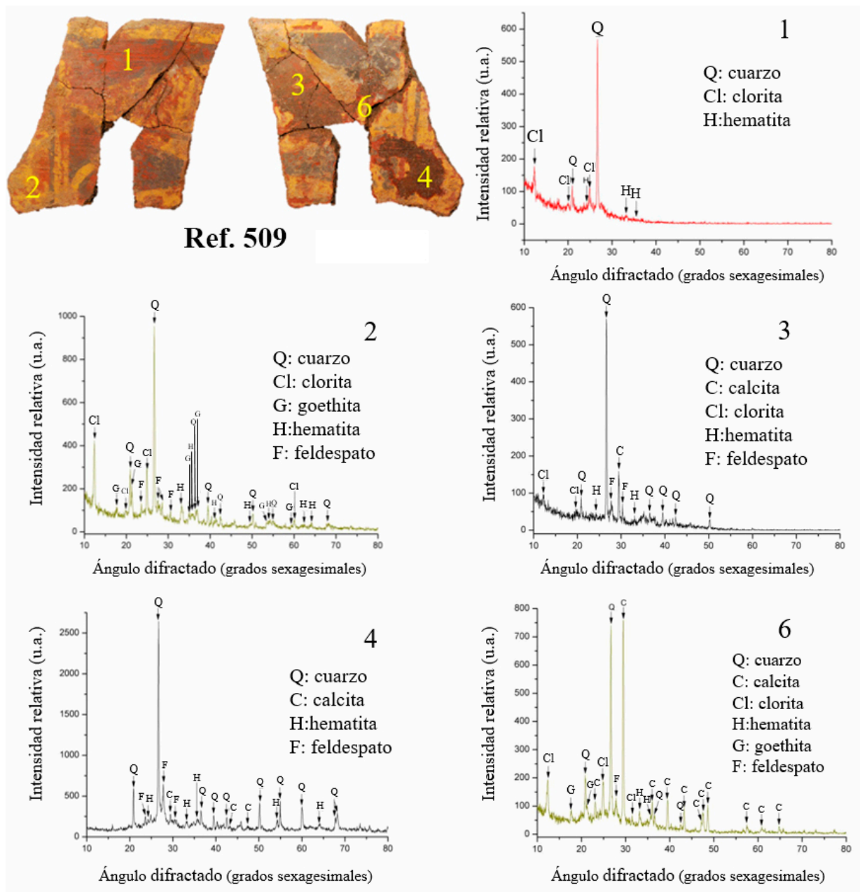
FIG. 2. Imagen de las muestras procedentes del yacimiento del Cerro Borreguero (Zalamea de la Serena), donde se señalan los puntos donde se han efectuado los análisis, así como los difractogramas.
