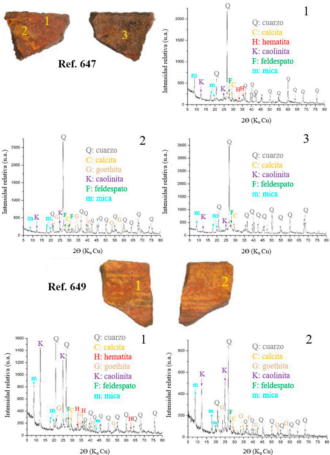
FIG. 12. Muestras procedentes del yacimiento de San Martín de Ledesma (Salamanca) donde se señalan los puntos donde se han efectuado los análisis y los difractogramas resultantes.
