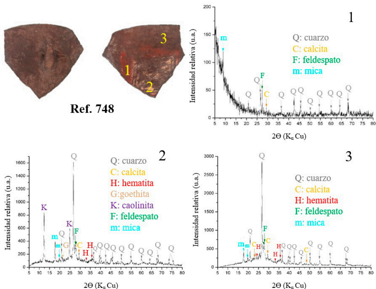
FIG. 6. Muestra procedente del yacimiento de Sanchorreja (Ávila) donde se señalan los puntos donde se han efectuado los análisis y los difractogramas resultantes.
