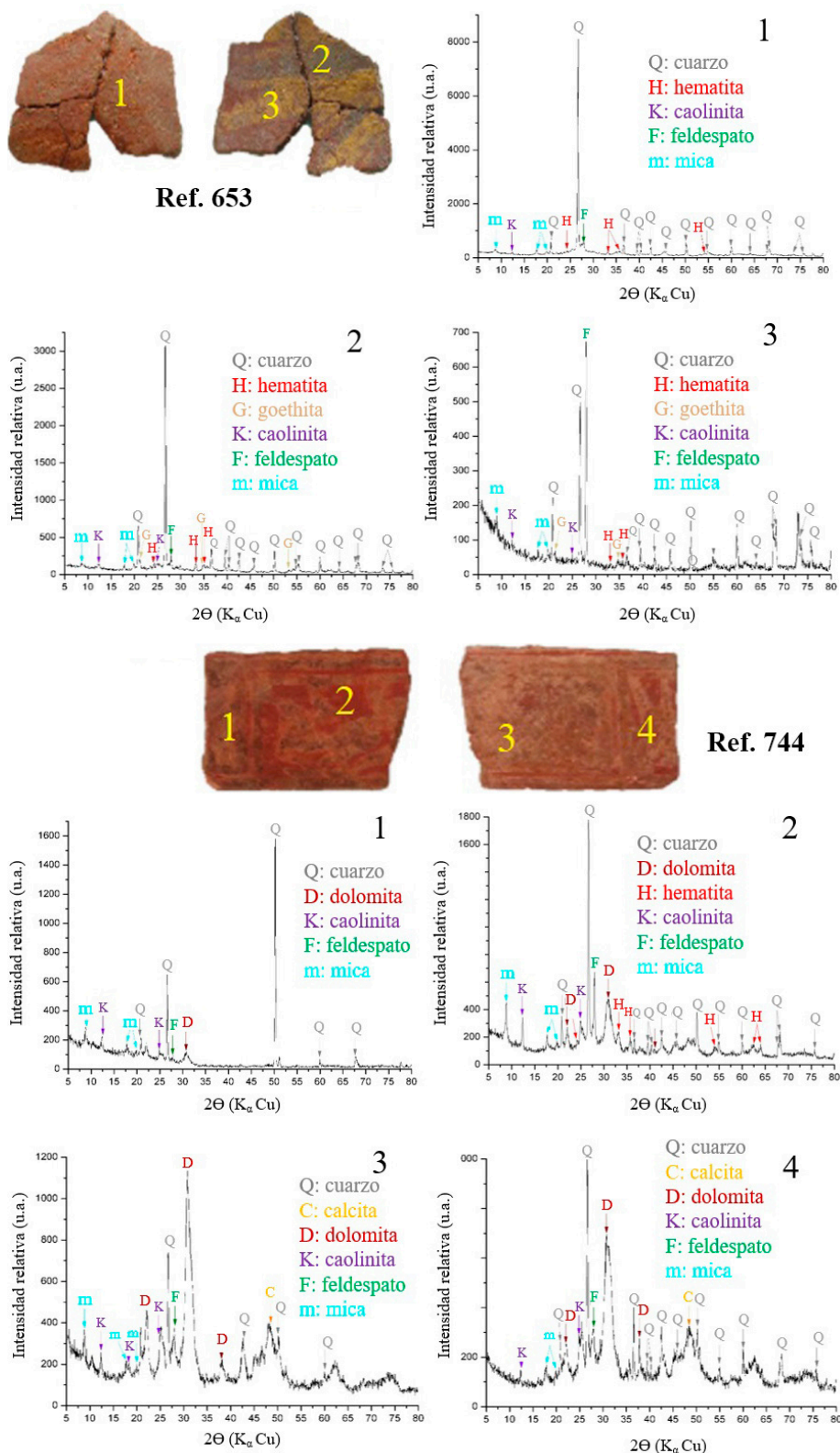
FIG. 7. Muestras procedentes tanto de la necrópolis como del Cerro del Castillo de Medellín (Badajoz) donde se señalan los puntos donde se han efectuado los análisis y los difractogramas resultantes.
