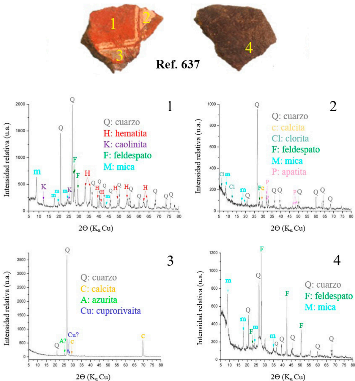
FIG. 5. Muestras procedentes del yacimiento de La Aldehuela (Zamora) donde se señalan los puntos donde se han efectuado los análisis y los difractogramas resultantes.
