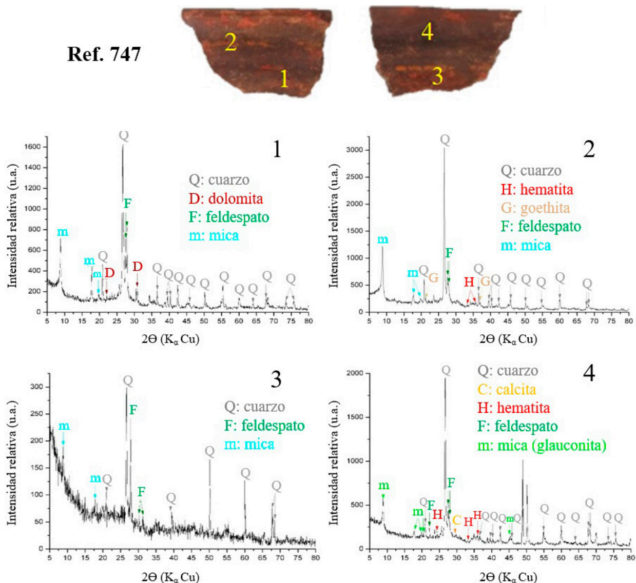
FIG. 10. Muestras procedentes del yacimiento de la Casa del Carpio (Belvís de la Jara, Toledo) donde se señalan los puntos donde se han efectuado los análisis y los difractogramas resultantes.
