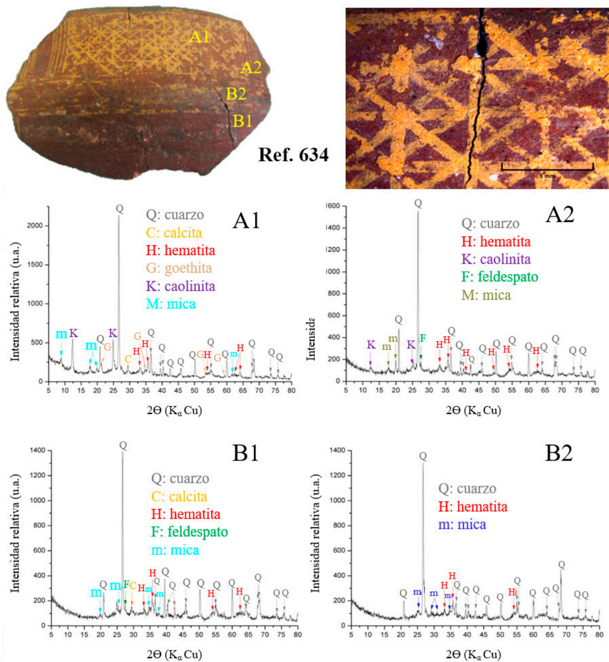
FIG. 9. Muestra procedente del yacimiento de Sima de Cabeza de la Fuente (Cuenca) donde se señalan los puntos donde se han efectuado los análisis y los difractogramas resultantes.
