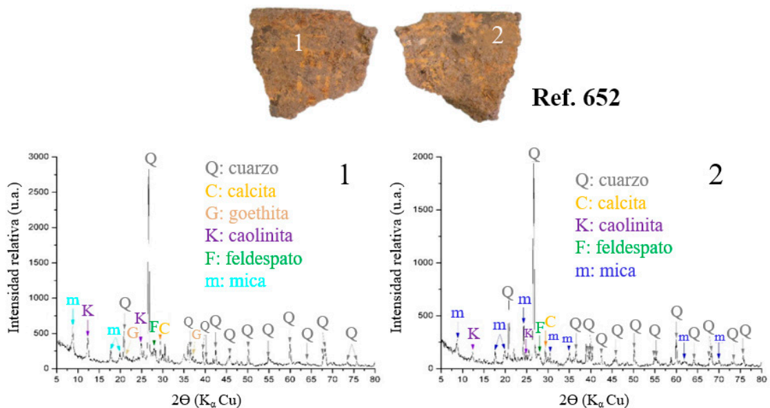
FIG. 14. Muestra procedente del yacimiento de Cerro de San Vicente (Salamanca) en la que se señalan los puntos donde se han efectuado los análisis y los difractogramas resultantes.
