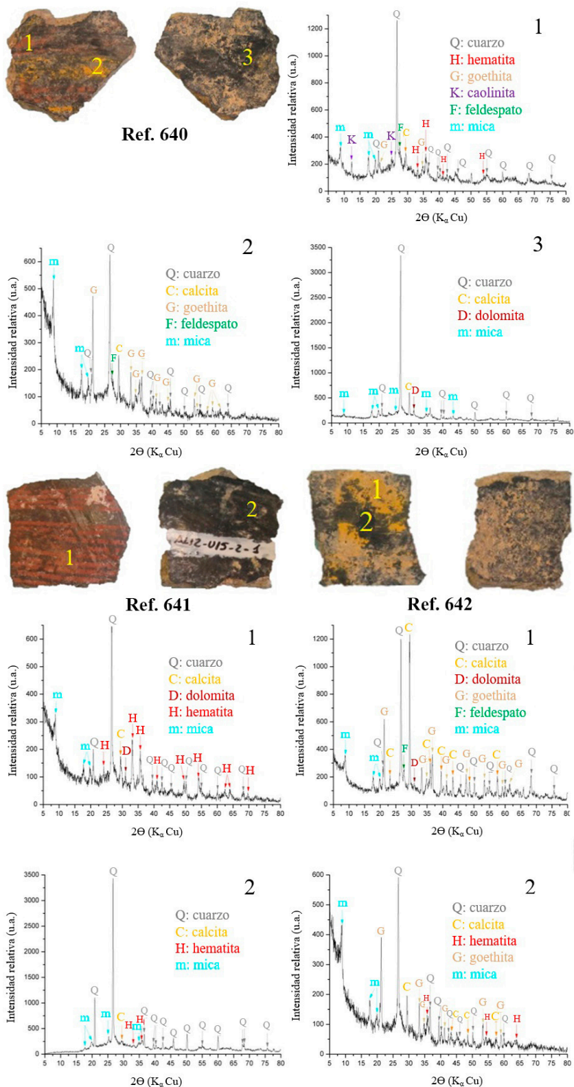
FIG. 8. Muestras procedentes del yacimiento de Alarcos (Ciudad Real) donde se señalan los puntos donde se han efectuado los análisis y los difractogramas resultantes.
