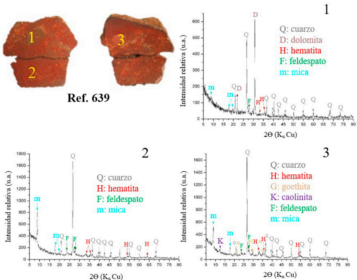
FIG. 11. Muestras procedentes del yacimiento de Santarém (Portugal) donde se señalan los puntos donde se han efectuado los análisis y los difractogramas resultantes.
