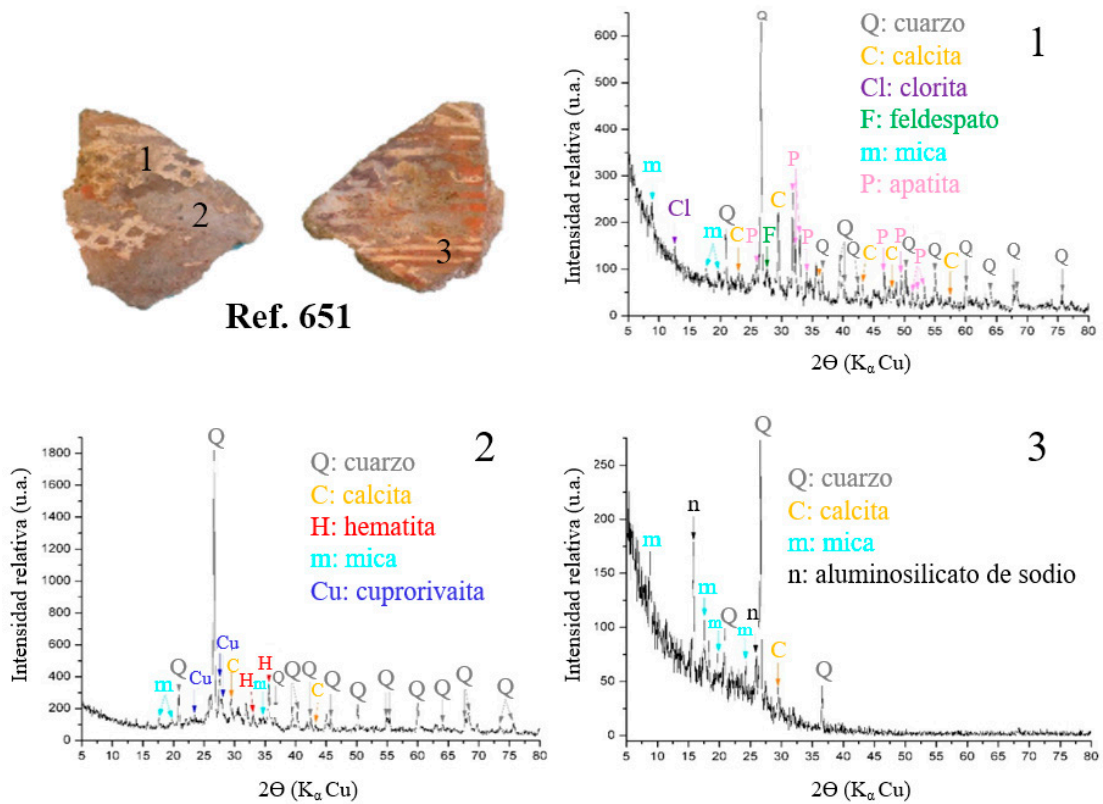
FIG. 13. Muestras procedentes del yacimiento de Cerro de San Pelayo (Martinamor, Salamanca) donde se señalan los puntos en los que se han efectuado los análisis y los difractogramas resultantes.
