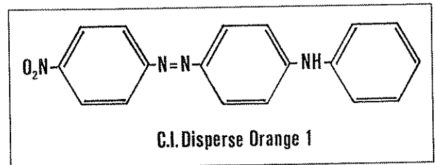
Figura 1. Estructura química del colorante azodisperso CI Disperse Orange 1.
