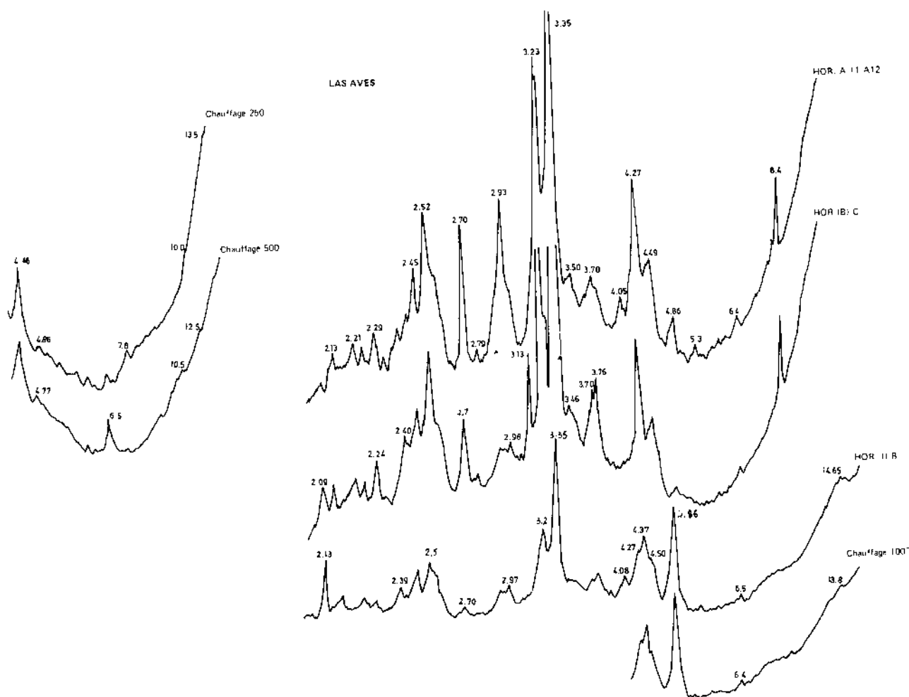
FIG. 4. — « Profil Las Aves ». Diagrammes de diffraction de rayons X (Sol total).
