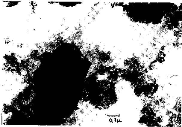
FIG. 5. — Microscopie électronique. Profil Las Aves. Hor. IIB. Imogolite.
