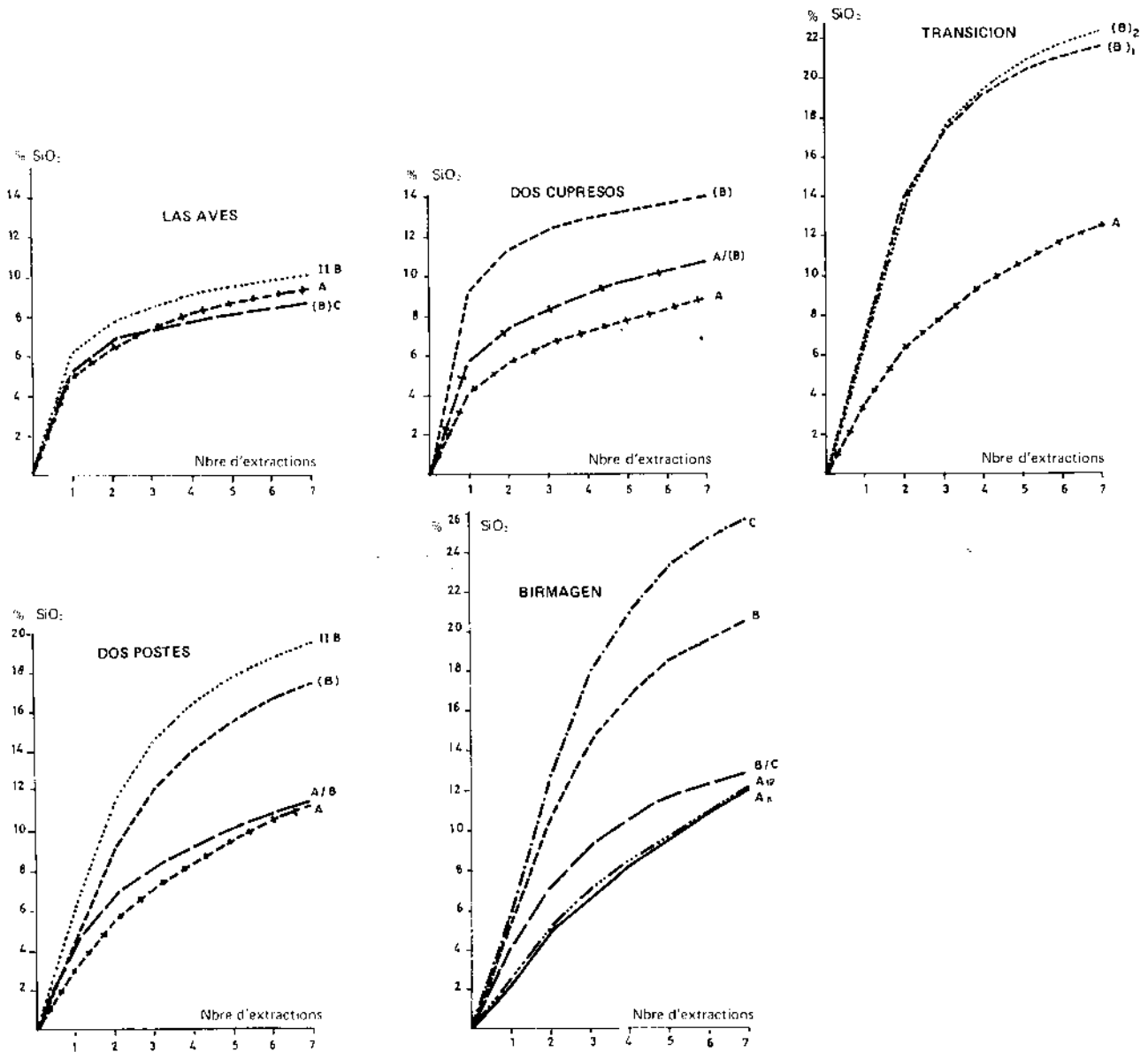
FIG. 1. — Courbes cumulatives de dissolution : SiO 2
