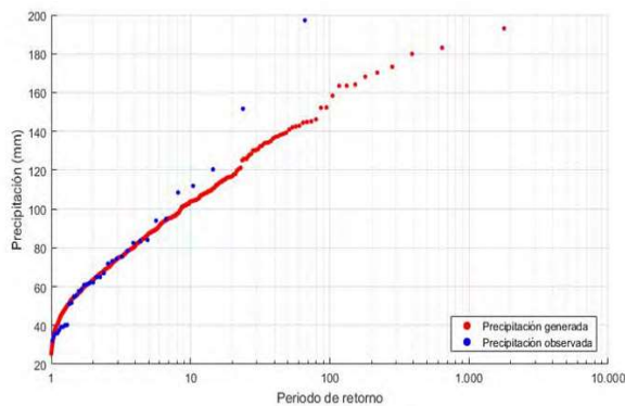
Fig. 2. Función de distribución empírica de la lluvia diaria máxima anual sobre el grid 3717 Fig. 2. Plotting positions of anual máxima daily rainfall.
