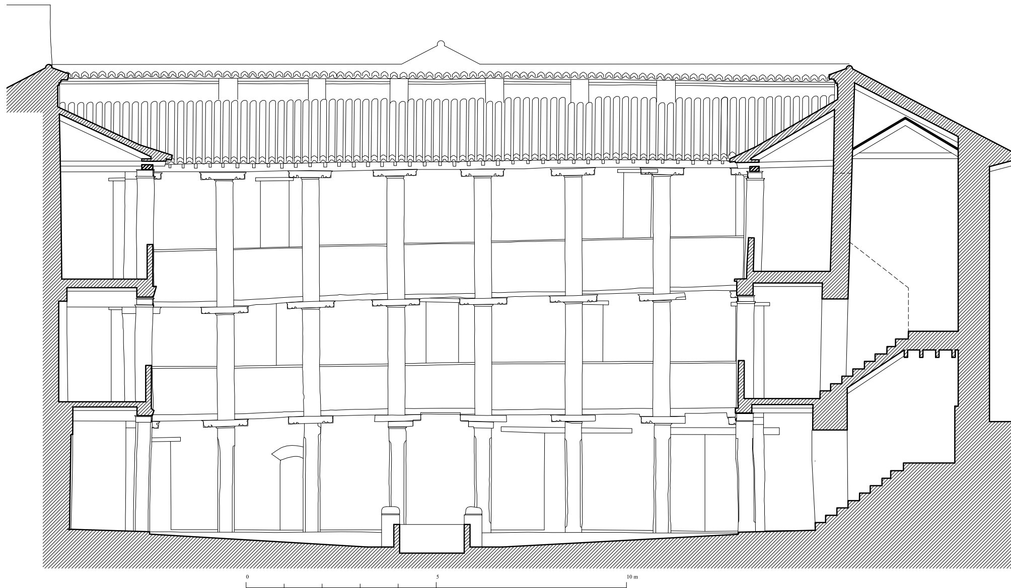
CORRAL DEL CARBON (Funduq al-Yadid). GRANADA. SECCION TRANSVERSAL ESCUELA DE ESTUDIOS ARABES. CSIC. noviembre 1994. A. ALMAGRO / arq. I. ZUÑIGA / arq. bc.
