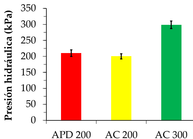
Figura 2. Presiones registradas por los transductores en los aspersores de impacto de cada tratamiento.
