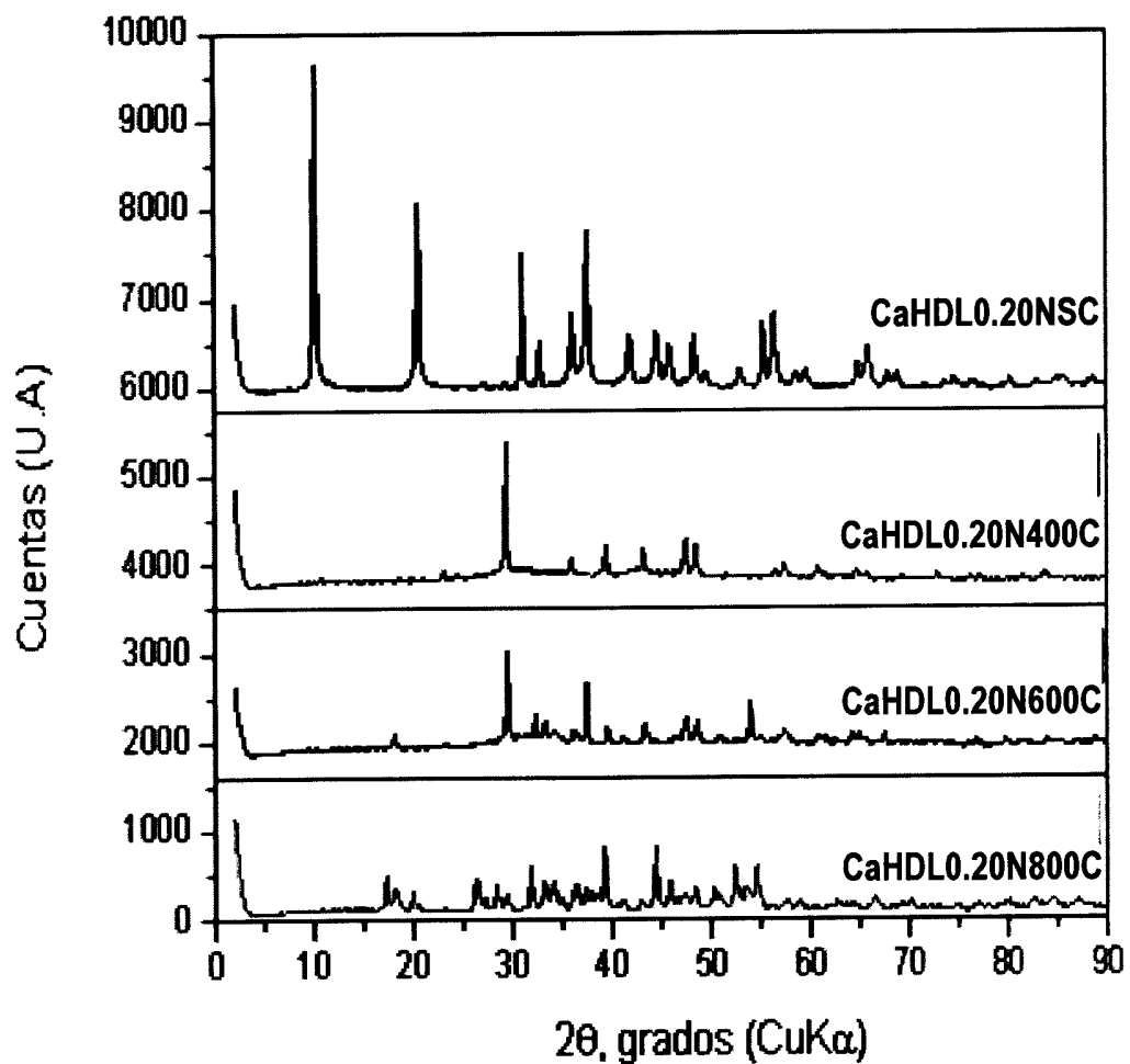
Figura 1. DRX del HDL de Ca calcinado a diferentes temperaturas.
