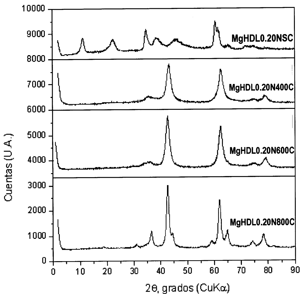
Figura 2. DRX del HDL de Mg calcinado a diferentes temperaturas.
