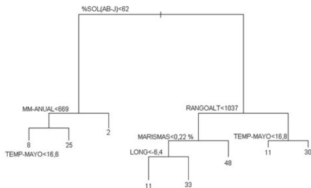
Figura 2. Árbol de regresión (modelo generalizado aditivo) mostrando los principales factores ambientales (ramificaciones) responsables de la frecuencia de aparición de la Cigüeñuela en España. Los valores de las puntas del árbol de regresión ilustran la ocupación de cuadrículas UTM 10x10 km dentro de bloques UTM de 50x50 km (expresado en %). La longitud de las ramas es proporcional a la importancia cuantitativa de cada variable explicando la distribución de la especie en España. %SOL(AB-J): insolación durante Abril-Junio (% de horas con el cielo despejado); MM-ANUAL: precipitación anual (en mm); TEMP-MAYO: temperatura media durante el mes de Mayo (en °C); LONG: longitud (en grados); MARISMAS: porcentaje de superficie de las cuadrículas UTM de 10x10 km cubiertas por marismas; RANGOALT: rango altitudinal de las cuadrículas UTM 10x10 km (en m). Análisis efectuado a partir de los datos del Atlas de las Aves de España (2003).
