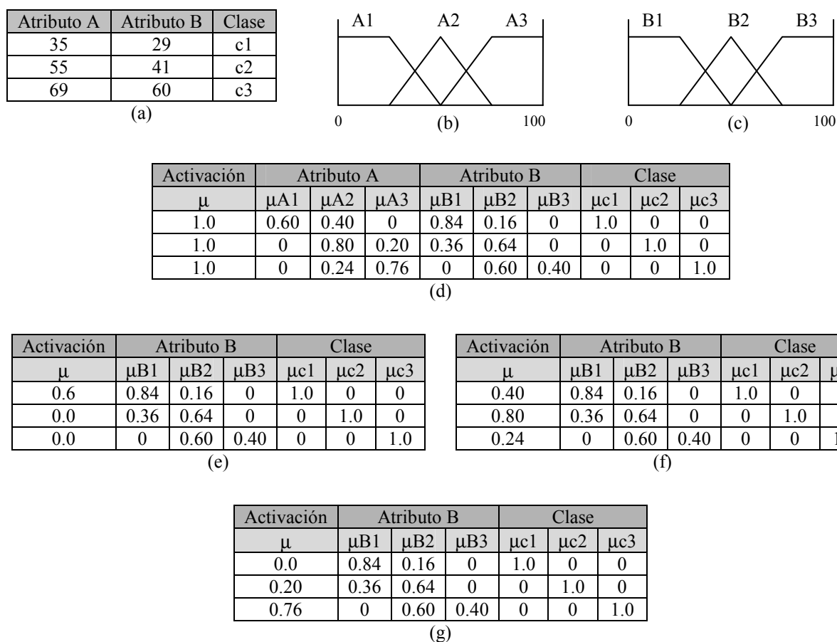
Figura 2: (a) Conjunto de datos original; (b,c) Funciones de pertenencia de los atributos A y B; (d) Conjunto de datos difusos; (e,f,g) Subconjuntos de datos difusos para los valores A1, A2 y A3 del atributo A.
