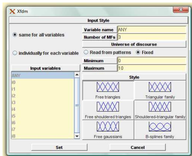
Figura 7: Configuración de las variables de entrada.
