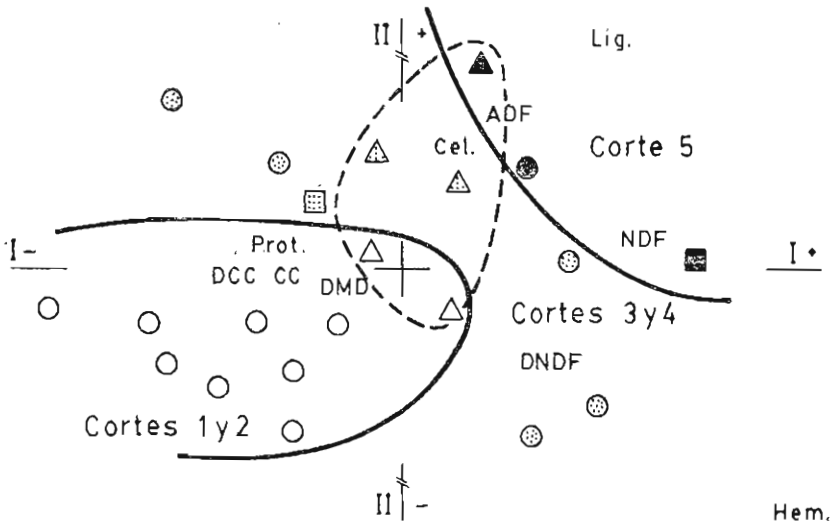
Fig. 3.—Ordenación de las muestras de Anthyllis utilizando como variables los resultados analíticos. Símbolos: círculos A. lotoides , triángulos A. vulneraria y cuadrados A. cornicina ; los cortes se indican mediante distintas tramas.
