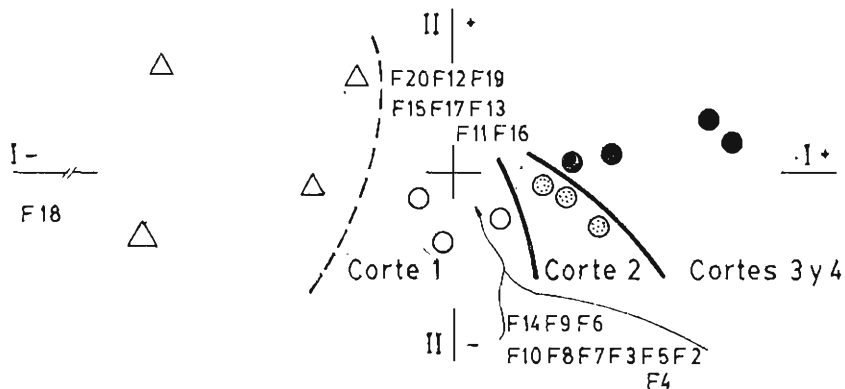
Fig. 11.—Ordenación de las muestras de Poa utilizando como variables 19 valores de reflectancia. Símbolos: círculos P. pratensis y triángulos P. bulbosa ; los cortes se indican mediante distintas tramas.
