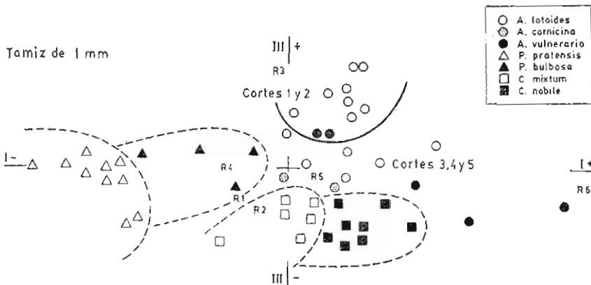
Fig. 5.—Ordenación general de las muestras, molidas a través de tamiz de 1 mm., utilizando como variables 6 valores de reflectancia.
