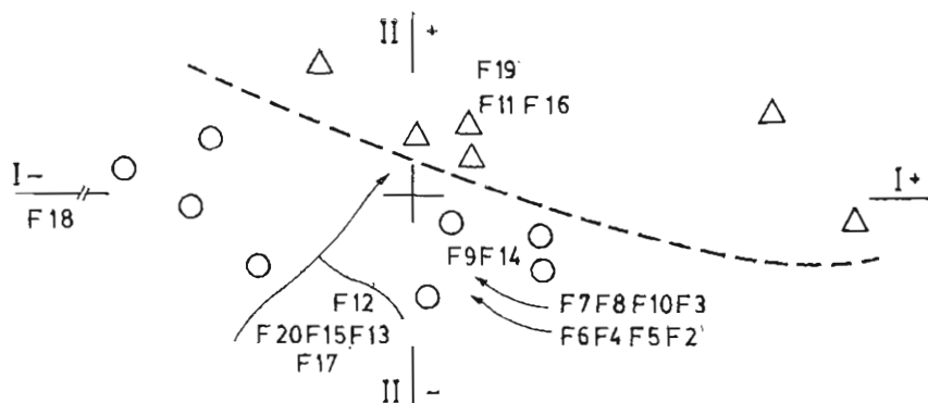
Fig. 13.—Ordenación de las muestras de Chamaemelum utilizando como variables 19 valores de reflectancia. Símbolos: círculos C. nobile y triángulos C. mixtum .
