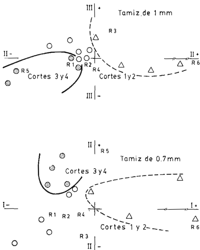
Fig. 7.—Ordenación de las muestras de Poa , de distinta granulometría, utilizando como variables 6 valores de reflectancia. Símbolos: círculos P. pratensis y triángulos P. bulbosa ; los cortes se indican mediante distintas tramas.
