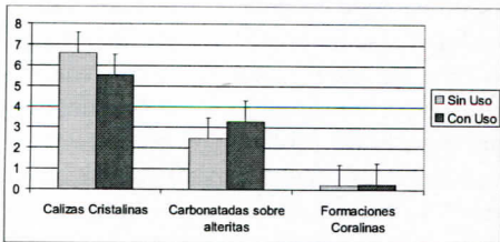
Figura 4. Estimación de las posibilidades de pérdida de suelo (medias y desviaciones típicas) según los grandes grupos litológicos donde éstos se desarrollan.
