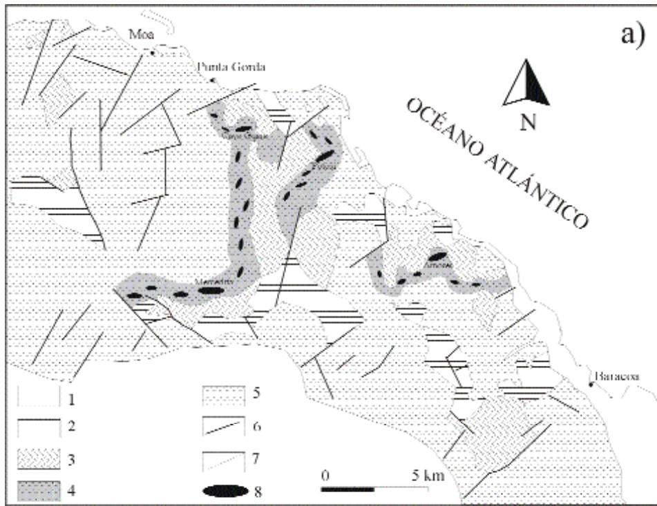
Figura 2. a) Mapa geológico (adaptado a partir de Nagy et al., 1976) y localización de los principales depósitos de cromita dentro del Macizo Moa-Baracoa. 1) Rocas sedimentarias post-orogénicas, 2) rocas volcánicas Cretácicas, 3) gabros, 4) Moho Transition Zone (harzburgitas, dunitas, peridotitas “impregnadas”, sills de gabros, diques de gabros y de pegmatoides gabroicos), 5) harzburgitas, 6) falla, 7) contacto tectónico, 8) depósitos de cromita. b) Propuesta de columna sintética ideal para el Macizo Ofiolítico Moa-Baracoa, reconstruida a partir de datos propios y bibliográficos (Thayer, 1942; Guild, 1947; Ríos y Cobiella, 1984; Fonseca et al., 1985, 1992; Torres, 1987; Murashko y Lavandero, 1989; Iturralde-Vinent, 1996). La dimensión no está a escala. 1) Basaltos y cherts, 2) diques de diabasa, 3) gabros isotrópico, 4) gabros bandeado, 5) harzburgitas y dunitas, 6) harzburgitas, 7) sills de gabro, 8) diques de gabros y pegmatoides gabroicos, 9) cromititas.
