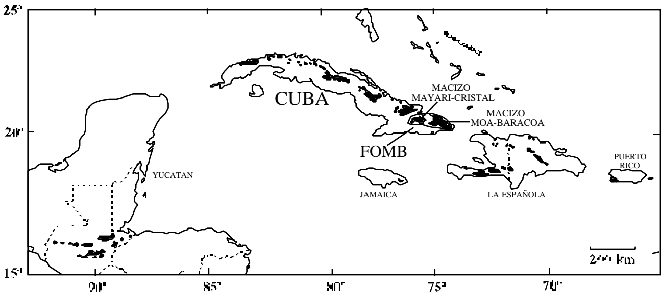
Figura 1. Principales afloramientos de rocas ofiolíticas en Cuba y en el Caribe noroccidental (modificado de Wadge et al., 1983). Nótese la ubicación de la Faja Ofiolítica Mayarí-Baracoa (FOMB) en el extremo oriental de la Isla de Cuba.
