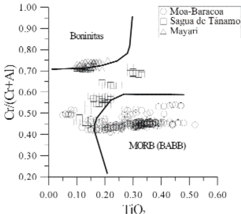
Figura 7. Cr/(Cr+Al) respecto al contenido de TiO_2 en las cromitas de la Faja Ofiolítica Mayarí-Baracoa. Los campos tipo boninitas y MORB son de Arai (1992).
