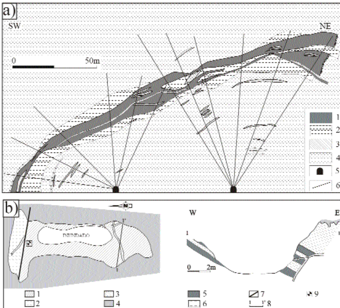
Figura 4. a) Perfil, a partir de un perfil de sondeos, a través de un lente del yacimiento Mercedita (distrito Moa-Baracoa). 1) cromititas, 2) dunitas, 3) sills de gabro, 4) principalmente harzburgitas, 5) estación de sondeos, 6) sondeos. b) Corte geológico de una cantera de explotación del yacimiento Casimba (distrito Mayarí). 1) Cromitites y dunitas, 2) harzburgitas, 3) diques de piroxenita, 4) laterites, 5) cromititas, 6) dunitas, 7) falla, 8) perfil, 9) pozo.
