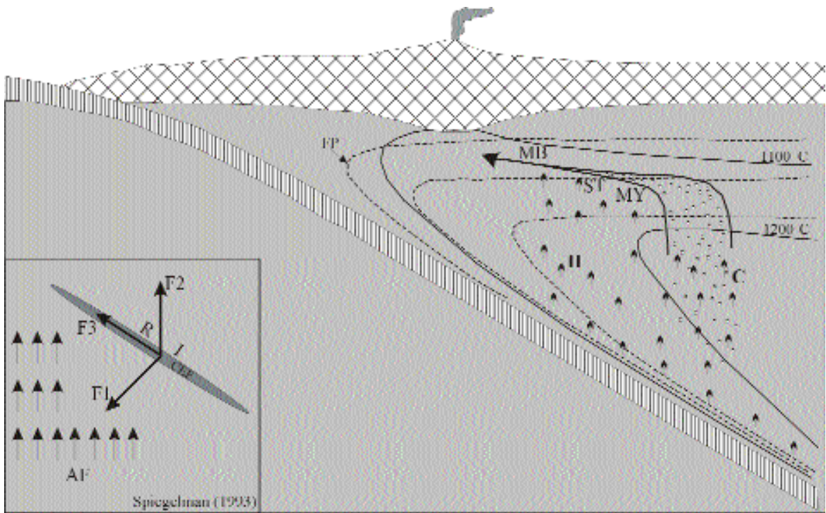
Figura 8. Modelo genético para la formación de las cromititas de la Faja Ofiolítica Mayarí-Baracoa (modificado de Proenza et al., 1999a) (ver texto para discusión). MB, cromititas del distrito Moa-Baracoa; ST, cromititas del distrito Sagua de Tánamo; MY, cromititas del distrito Mayarí; H, fundidos fuertemente hidratados; C, fundidos calcoalcalinos. En el modelo de Spiegelman (1993): FP, flujo plástico; AF, aporte de fundido; CEF, canales de expansión de fundidos; RI, región impermeable; F1, presión de compactación; F2, fuerza ascensional; F3, velocidad del fundido.
