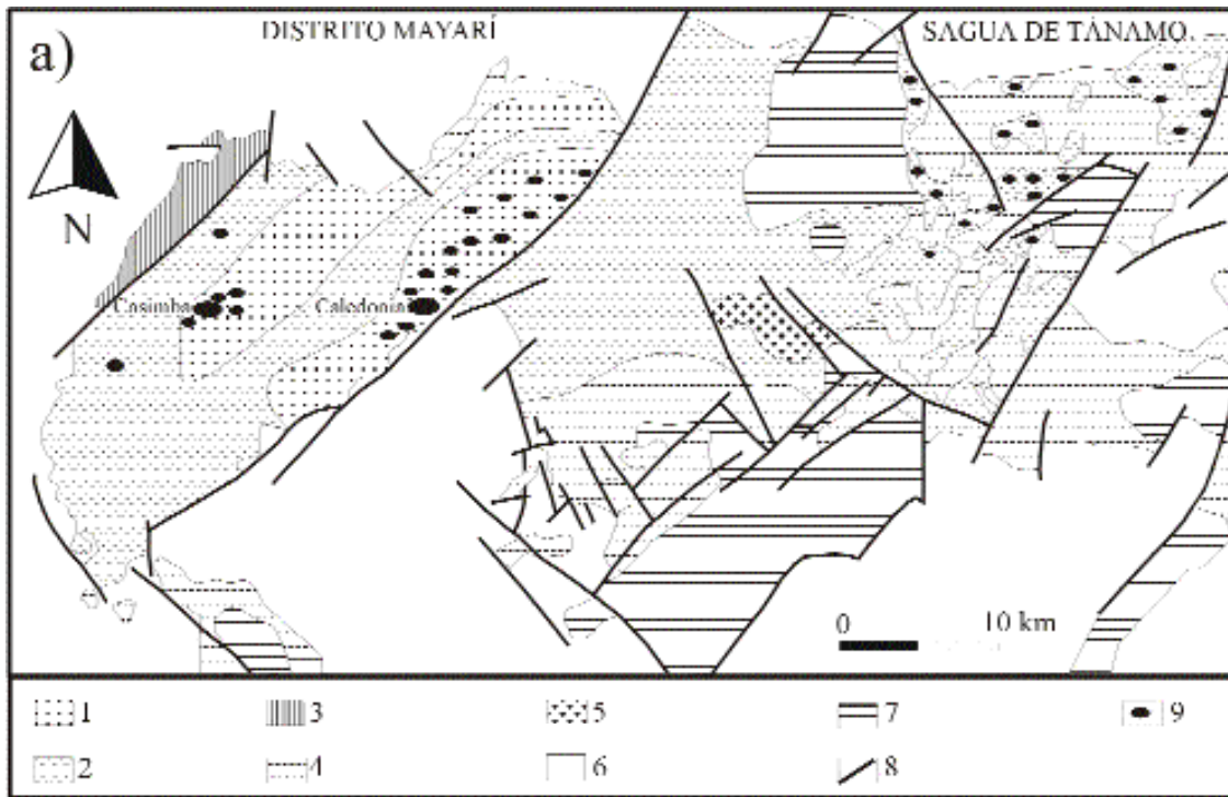
Figura 3 a) Mapa geológico del Macizo Mayarí-Cristal y localización de los principales depósitos de cromita de los distritos de: 1) Sagua de Tánamo y 2) Mayarí (modificado de Kravchenko y Vázquez, 1985; Nekrasov et al., 1989). 1) Dunitas y harzburgitas, 2) harzburgitas, 3) gabros y diques de diabasa, 4) zona de melange ofiolítico, 5) melange “La Corea”, 6) rocas sedimentarias post-orogénicas, 7) rocas volcánicas, 8) falla, 9) depósitos de cromita. b) Propuesta de columna sintética ideal para el Macizo Ofiolítico Mayarí-Cristal, reconstruida a partir de datos propios y bibliográficos (Thayer, 1942; Fonseca et al., 1985, 1992; Nekrasov et al., 1989; Murashko y Lavandero, 1989; Navarrete y Rodríguez, 1991; Iturralde-Vinent, 1996). La dimensión no está a escala. 1) Diques de diabasa, 2) gabros (?), 3) harzburgitas y dunitas, 4) harzburgitas, 5) diques de piroxenita, 6) cromititas.
