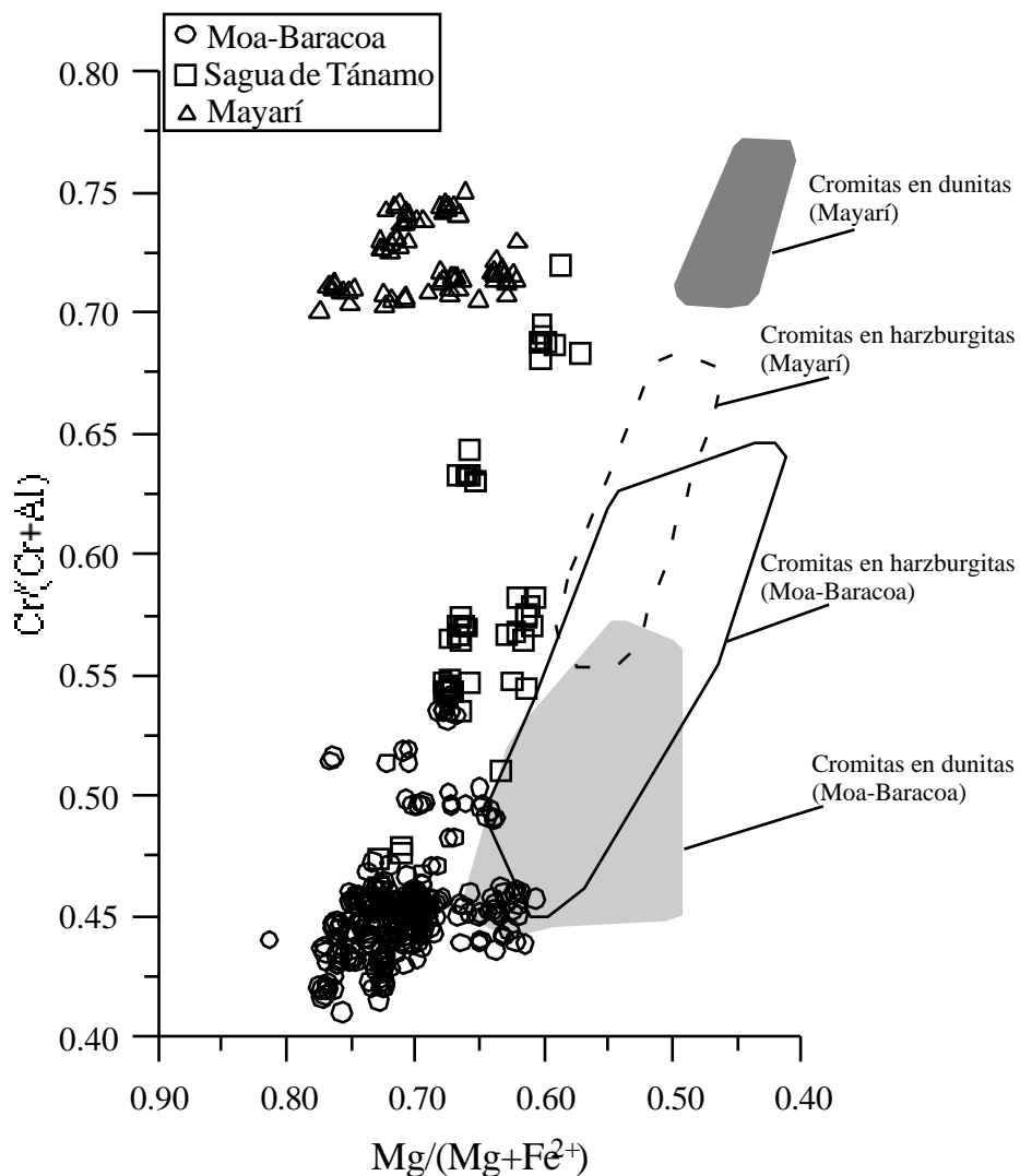
Figura 6. Cr/(Cr+Al) respecto a Mg/(Mg+Fe^{2+}) en las cromitas de la Faja Ofiolítica Mayarí-Baracoa. A manera de comparación también se muestra la composición química de las cromitas accesorias en las dunitas y harzburgitas.
