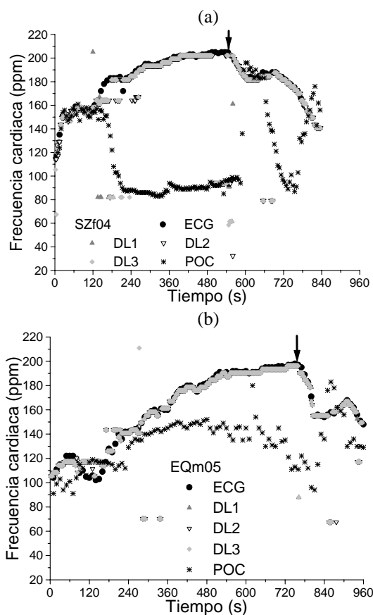
Fig.5.- Frecuencia cardiaca (pulsaciones por minuto, ppm) obtenida en una atleta (a, SZf04) y un atleta (b, EQm05) en una prueba de esfuerzo con electrocardiografía (ECG), un pulsioxímetro comercial (POC) y nuestro sistema con tres diodos láser (DL1, DL2 y DL3).
