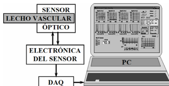
Fig.1.- El sistema de medida está compuesto por el sensor óptico basado en diodos láser del infrarrojo cercano, fijado al extremo de un dedo (lecho vascular pulsátil), electrónica del sensor y un ordenador personal (PC) con la tarjeta de adquisición de datos (DAQ) y los programas de adquisición y procesamiento.
