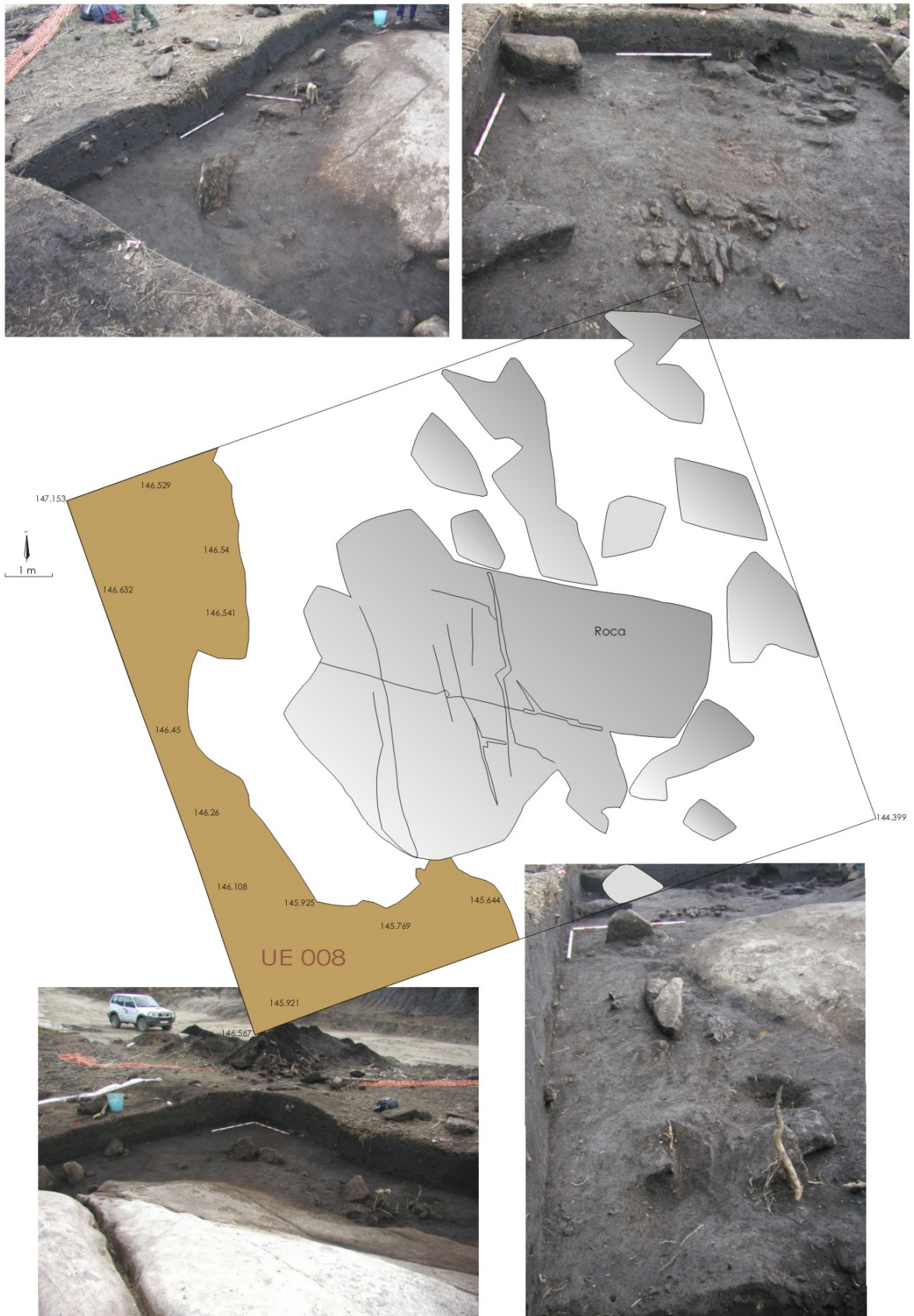
Figura 18. Planimetría e vistas da UEDEV01008 nas UR 22, 23, 32, 42 y 43
