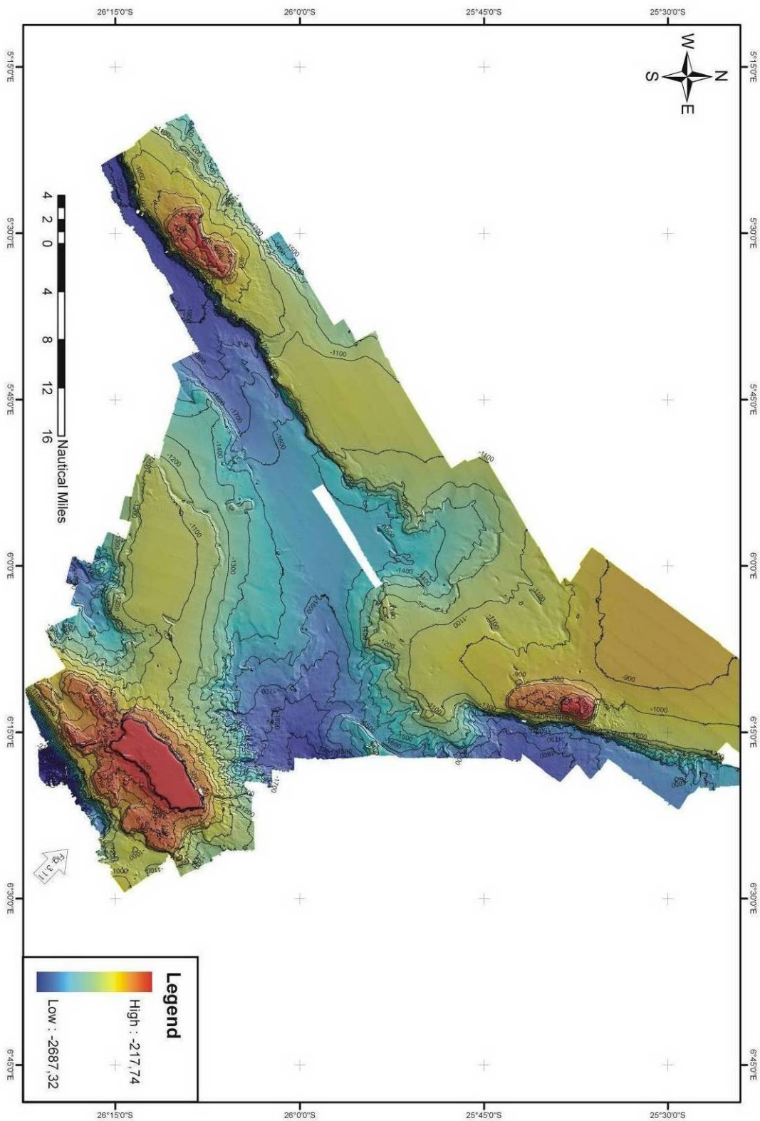
Figura 3.10: Mapa batimétrico de los montes Valdivia Centro, Valdivia Oeste y Valdivia Sur / Bathymetric map of the Valdivia Central, Valdivia West and Valdivia South Seamounts.
