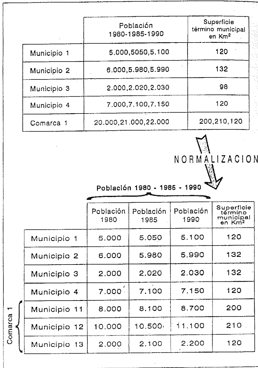
FIGURA 2.—Normalización de relaciones
