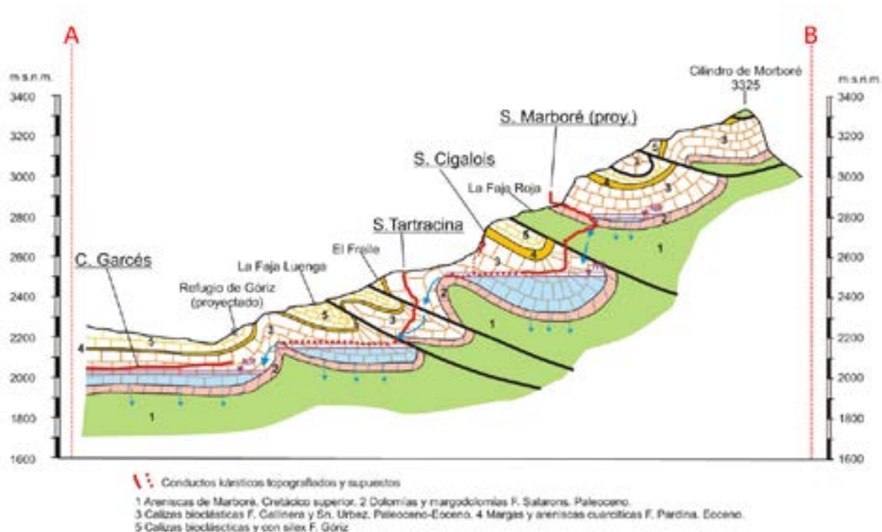
Figura 6.10. Corte geológico siguiendo el perfil A-B en la Figura 11. Sobre el corte se muestra la proyección de las simas a través de las cuales se inyectaron los diferentes trazadores. La línea roja, a tramos discontinua, indica la posible trayectoria de los trazadores con el flujo subterráneo a través del sistema kárstico.
