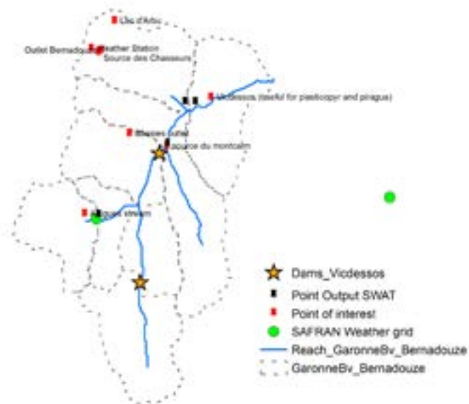
Figura 8.3. Principales elementos de la modelización hidrológica de la turbera de Bernadouze, en el Alto Vicdessos. (Fuente: elaboración propia.)
