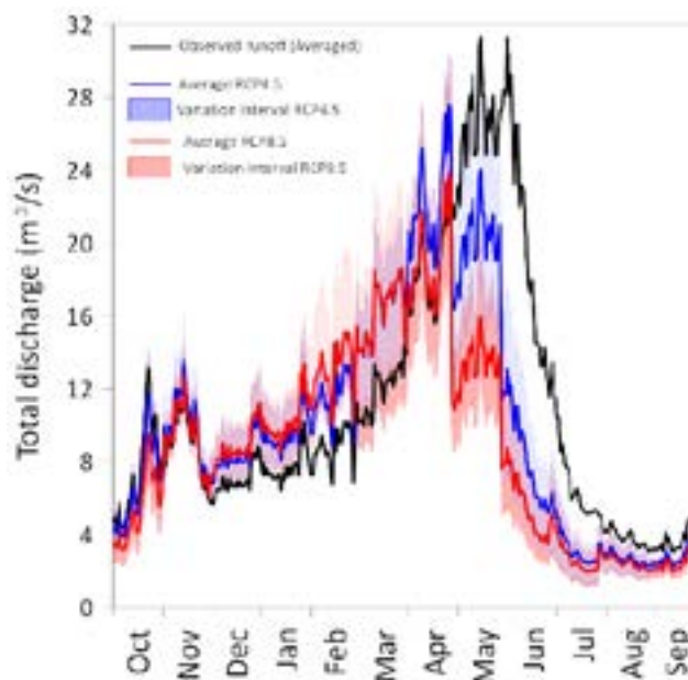
Figura 6.6. Variación estacional de la descarga total del río Ara, para el periodo de control (1961-2005) como para el periodo 2071-2100 teniendo en cuenta los escenarios de cambio climático RCP 4.5 y RCP 8.5 simulados por los diferentes modelos climáticos.
