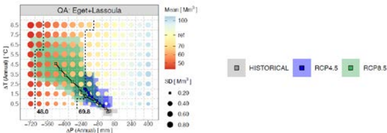
Figura 4.3: Superficie de respuesta que caracteriza la sensibilidad de las entradas naturales totales a los lagos-embalses a las perturbaciones climáticas. Las curvas representan posibles trayectorias desde el periodo actual hasta el final del siglo, muestreadas cada 10 años con los escenarios RCP4.5 (azul) y RCP8.5 (verde). Cada punto es representativo de un periodo consecutivo de 20 años (media de 6 proyecciones climáticas). Las zonas en azul y verde representan la dispersión de las proyecciones del clima del proyecto CLIMPY. Los límites de las zonas críticas para los usos en relación con el cambio climático se identifican con líneas en negro.
