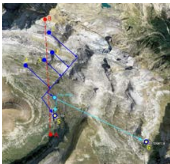
Figura 6.9. Puntos de inyección de trazador en el ensayo de agosto 2019 (1: Sima Marboré; (2) Sima Cigaloís; (3) Sima Tartracina; (4) Sima-60), y puntos de descarga asociados a los manantiales Garcés (5) y Fuenblanca (6) La línea A-B marca la trayectoria del perfil geológico mostrado en la Figura 6.12.
