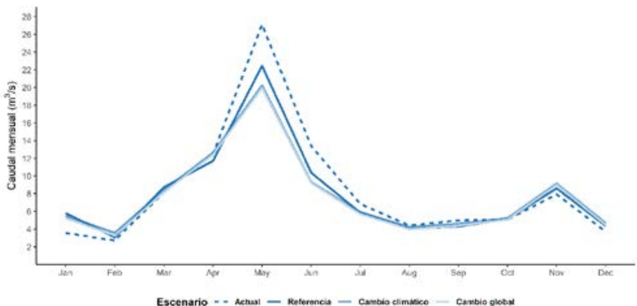
Figura 3.4. Cambio en el régimen mensual de caudal en la salida de la cuenca de Andorra (Borda Sabaté) en el año 2050 en el escenario Actual y en los escenarios Referencia, Cambio climático y Cambio global.
