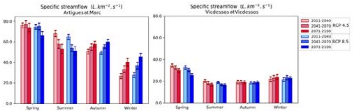
Figura 8.7. Caudal específico estacional medio en Artigues y Videssos para diferentes horizontes temporales y escenarios de emisión. Las barras rojas representan el escenario RCP 4.5 y las azules el escenario RCP 8.5. Primavera corresponde a los meses de Abril a Junio, verano de Julio a Septiembre, otoño de Octubre a Diciembre, e invierno de Enero a Marzo.
