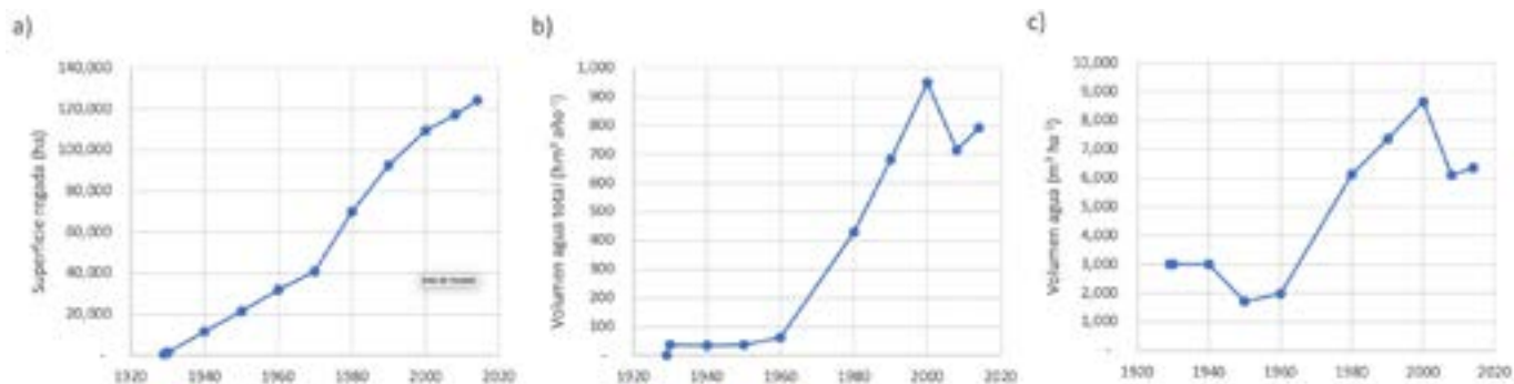
Figura 5.3. Evolución de la superficie regada (a), volumen de agua suministrado (b), y volumen de agua por unidad de superficie (c) en el sistema Riegos del Alto Aragón.
