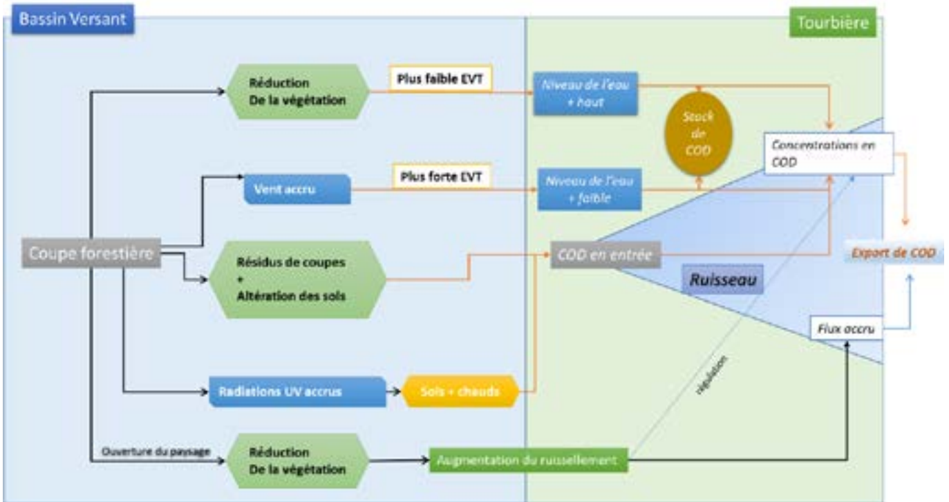
Figura 8.9. Esquema de las relaciones entre distintas variables hidro-geoquímicas potencialmente afectadas por una tala forestal en el entorno de una turbera. EVT: évapotranspiration; COD: carbone orgánico disuelto.
