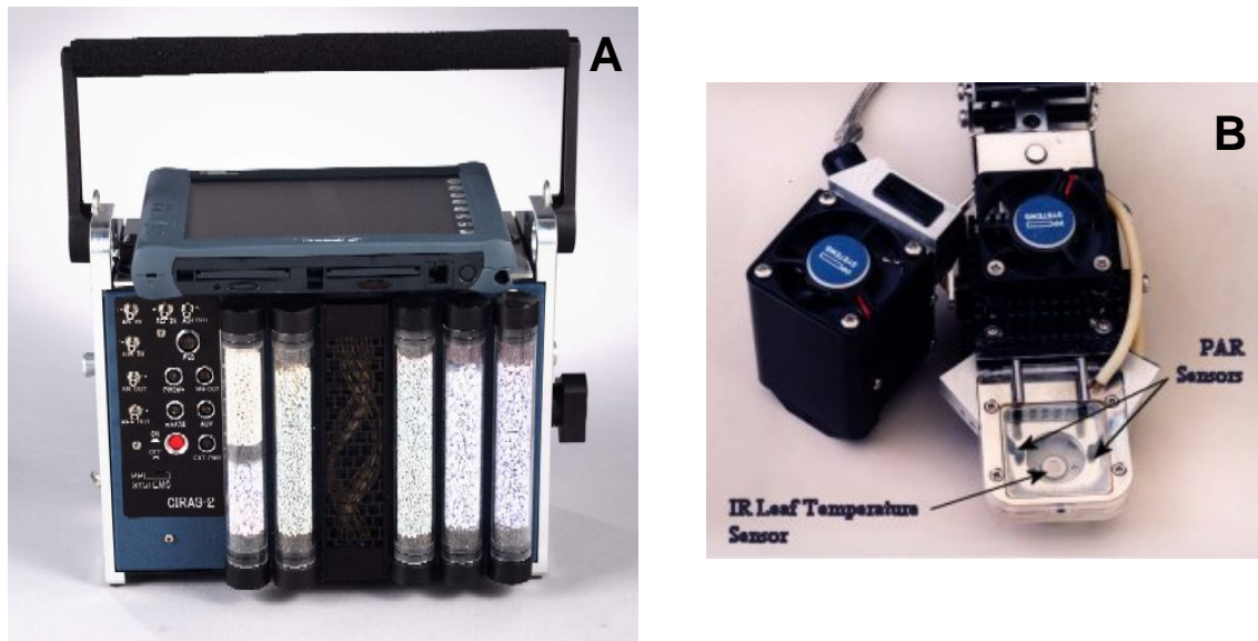
Fig 3.7. Imagen del IRGA Ciras 2 (A) y detalle de la cámara foliar que lleva adaptada para la medida en hojas in vivo (B). ( http://www.ppsystems.com )
