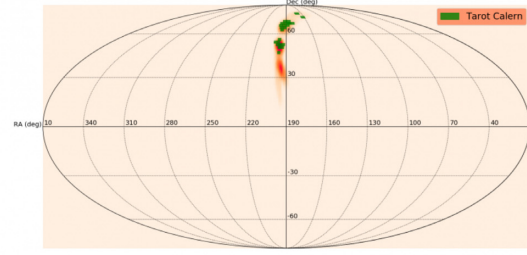
(d) S190915ak
