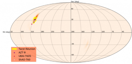
(f) S190718y
