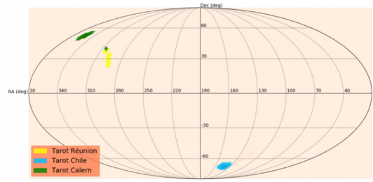
(d) S190727h
