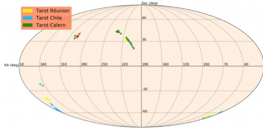
(e) S190720a
