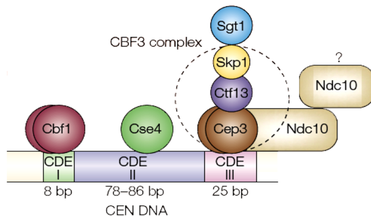
Figura I22. Organización de los 3 elementos funcionales (CDEI, CDEII y CDEIII) del centrómero puntual de S. cerevisiae y proteínas con las que interaccionan.
