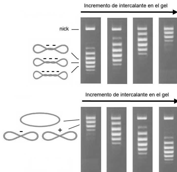
Figura M2. Esquema del efecto de un intercalante en la movilidad electroforética de distribuciones de Lk. En el panel de arriba, topoisómeros con superenrollamiento negativo ( \Delta W_r < 0 ) son más compactos y migran más rápido que el ADN relajado ( \Delta W_r = 0 ) o con cortes (nicks). Al añadir intercalante durante la electroforesis, se reduce T_w y estas moléculas de ADN covalentemente cerradas lo compensan incrementando W_r . En consecuencia migran más despacio. En el panel de abajo, topoisómeros cercanos a Lk^0 (distribución relajada, \Delta W_r = 0 ) migran cercanos al nick. Al añadir intercalante, se reduce T_w y estas moléculas de ADN lo compensan incrementando W_r , que en este caso pasa a ser W_r > 0 . En consecuencia, adquieren mayor velocidad en el gel.
