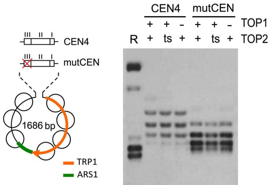
Figura R10. Distribuciones de Lk de los minicromosomas de 1686 pb, conteniendo CEN4 o mutCEN, en cepas de S. cerevisiae deficientes en topoisomerasas: JCW25 ( TOP1 TOP2 ), JCW26 ( TOP1 top2-ts ), JCW27 ( top1 TOP2 ).
