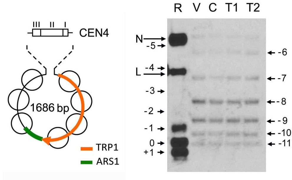
Figura R9. Topología del minicromosoma centromérico de 1686 pb extraído de células fijadas in vivo (V), extraído como cromatina nativa (C) y tras su incubación con topoisomerasa I (T1) y topoisomerasa II (T2). El mismo ADN desproteínizado y relajado se muestra en la primera calle (R).
