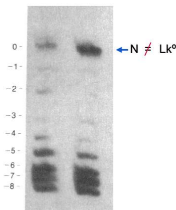
Figura D1. Electroforesis de ADN con la que Pederson et al (1986) concluyeron que la diferencia de enlace ( \Delta Lk=Lk-Lk^0 ) del minicromosoma TA1 es aproximadamente -7. Para ello, los autores consideraron incorrectamente que la posición de Lk^0 en el gel coincide con la del ADN circular covalentemente abierto o nicked (N).
