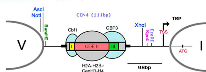
Figura R12. Mapa detallado de insertos del centrómero en minicromosomas de la generación 3 (1461 pb), generación 4 (1341 pb) y generación 5 (1286 pb). Se indica la posición de los nucleosomas I, V ó VI de TA1 y se indica la distancia entre el centrómero y el TSS del gen TRP1.
