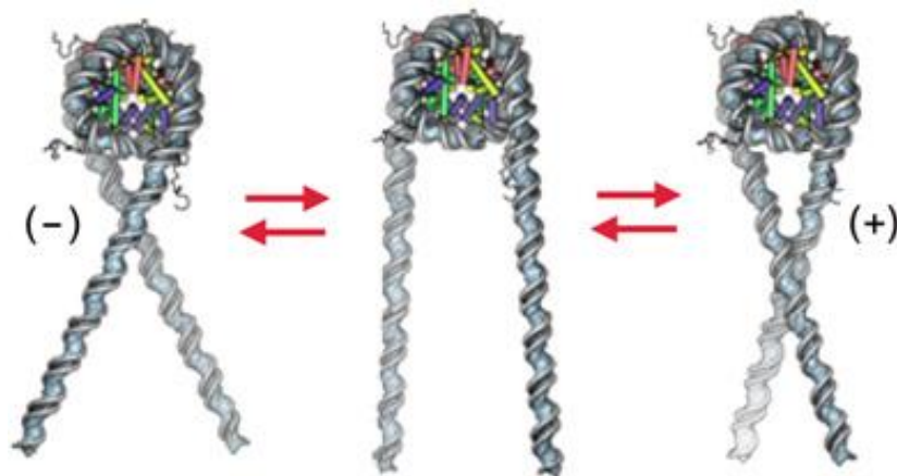
Figura I19. Los segmentos de entrada y salida del ADN en el nucleosoma pueden cruzarse en signo (-), tal como se describe en el complejo canónico o bien cruzarse en signo (+) debido a las fluctuaciones conformacionales de la cromatina.
