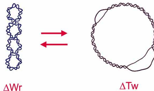
Figura I3. En un dominio cerrado de ADN con un valor de L_k constante, las deformaciones por W_r y por T_w pueden interconvertirse, L_k = T_w + W_r . El plásmido con notable superenrollamiento negativo ( \Delta W_r , izquierda) puede deformarse para abrir regiones de su doble hélice ( \Delta T_w , derecha).
