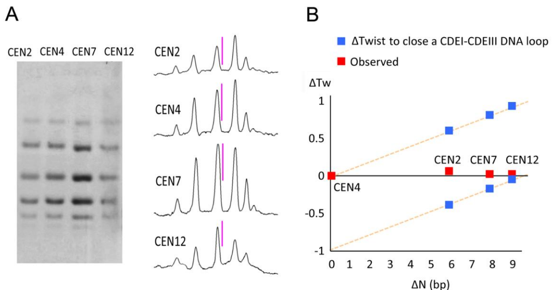
Figura R19. A. Electroforesis (agarosa 1.2%, cloroquina 0.6 \mu g/ml TBE, 70 V, 20 h) que muestra las distribuciones de Lk de los minicromosomas de 1341 pb con 4 centrómeros distintos. Los plots densitométricos revelan que las 4 distribuciones están centradas (eje rosa) en un mismo valor de Lk. B. Representación de los anteriores resultados experimentales (rojo) y de los cambios de Tw esperados (azul) en el caso de que cbf1 y CBF3 interaccionasen para cerrar un loop CDEI-CDEIII. \Delta N indica el número de pb de diferencia de los centrómeros respecto a CEN4.
