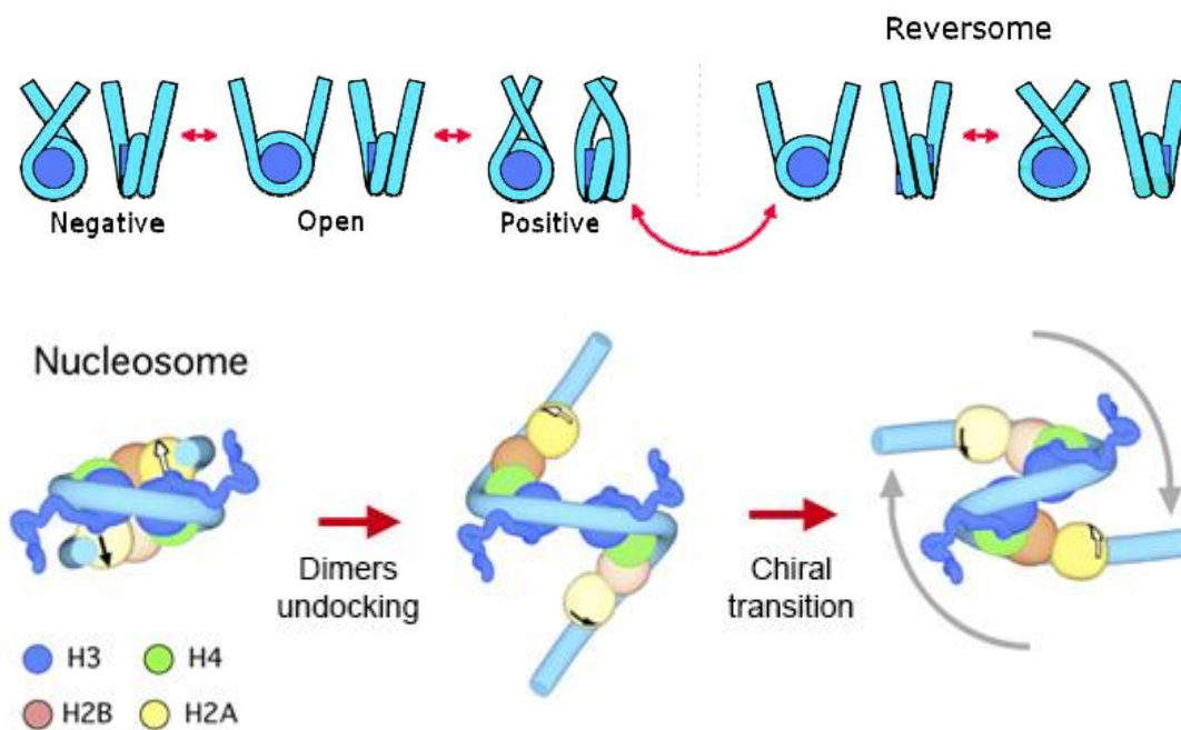
Figura I20. En la transición de nucleosoma a reversoma, la vuelta central que completa el ADN sobre el octámero de histonas pasa de levógira ( \Delta Wr < 0 ) a dextrógira ( \Delta Wr > 0 ). Esta transición se acompañaría de un cambio estructural del tetrámero (H3H4) 2 y una reorganización de los dímeros (H2AH2B).
