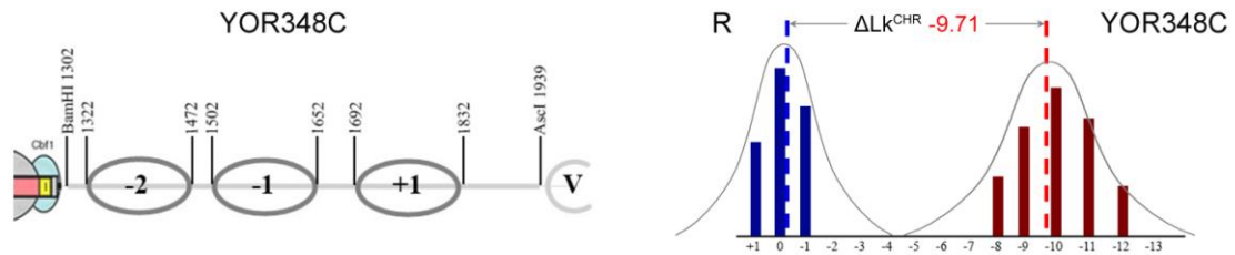
Figura R22. Posicionamiento de nucleosomas en los 11 segmentos de 630 pb (cromatina control y 10 promotores) insertados entre CEN4 y el nucleosoma V de TA1. Las diferencias de Lk de cada uno de estos 11 minicromosomas fijados in vivo a 28 °C respecto al ADN relajado in vitro se calculó con los histogramas de la derecha. Cada uno promedia 3 experimentos como los mostrados en las electroforesis de la figura previa.
