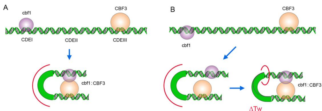
Figura R17. Distintas distancias entre CDEI y CDEIII implican que cbf1 y CBF3 quedan en fases rotacionales diferentes. En el caso de que cbf1 y CBF3 interaccionen (A), un aumento de longitud del segmento de doble hélice que los separa (CDEII) implicaría un ajuste mediante un cambio de twist ( \Delta Tw ) (B).
