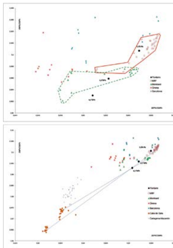
Fig. 10. Representación de los resultados de los análisis de isótopos de plomo de los brazaletes de Sebes (Flix, Tarragona) (véase Tab. 1) en relación a los materiales de otros yacimientos del I Hierro del Noreste de la Península Ibérica y mineralizaciones de la misma (I. Montero) (en color en la edición electrónica).
