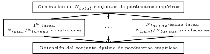
Figura 4.2: Diagrama de flujo del esquema de la paralelización en MPCOTool para métodos de fuerza bruta (barrido y Monte-Carlo).
