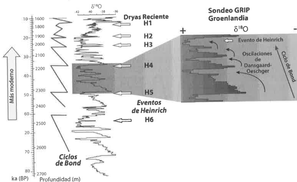
Figura 12.- Cambios climáticos rápidos reflejados en las variaciones del \delta^{18}O ‰ en el sondeo GRIP para el intervalo de 10 a 90 ka (según Bond et al. , 1993). Se representan también los ciclos de Bond, los eventos Heinrich y las oscilaciones Dansgaard-Oeschger (D-O). (Según Dansgaard et al. , 1993).
