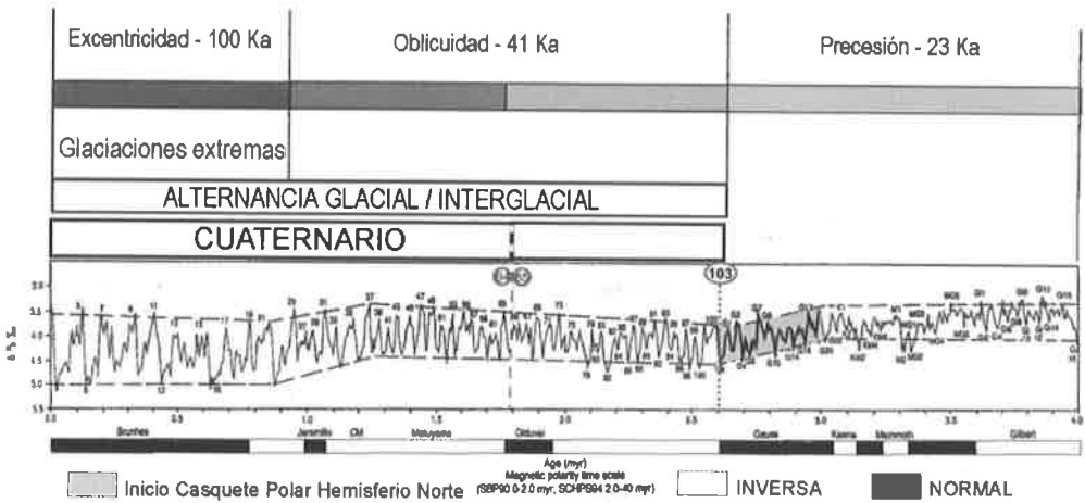
Figura 3.- Escala Isotópica Paleomagnética del Plioceno-Cuaternario. Registro isotópico del oxígeno para los últimos 4 Ma (según Shackleton, 1995; estos datos, junto con la escala paleomagnética, han sido recopilados por Patridge, 1997), con indicación de los ciclos o parámetros orbitales dominantes en un periodo determinado.
