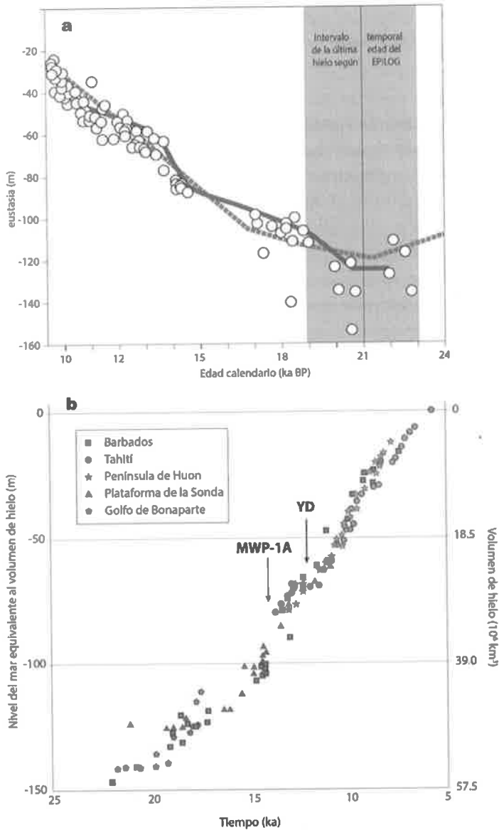
Figura 14.- (a) Curva teórica (línea discontinua) que muestra la subida del nivel del mar desde el nivel más bajo alcanzado durante el máximo del último periodo glaciario. En línea continua, curva del nivel del mar a partir de datos de los arrecifes de coral y los sondeos marinos (círculos) según el registro obtenido en los sedimentos. También se indica el intervalo temporal, franja gris, que se considera más probable para la máxima extensión del hielo en ambos hemisferios, según el consenso de EPILOG (Environmental Processes of the Ice Age: Land, Ocean, Glaciers). (Según Schneider et al., 2000). (b) Cambios en el volumen del hielo global desde el máximo glaciario hasta la actualidad basados en datos de la posición del nivel del mar en diferentes localidades, ajustado isostáticamente, según Lambeck et al., (2002). Clave: MWP (Melt Water Pulse), YD (Younger Dryas: Dryas reciente).
