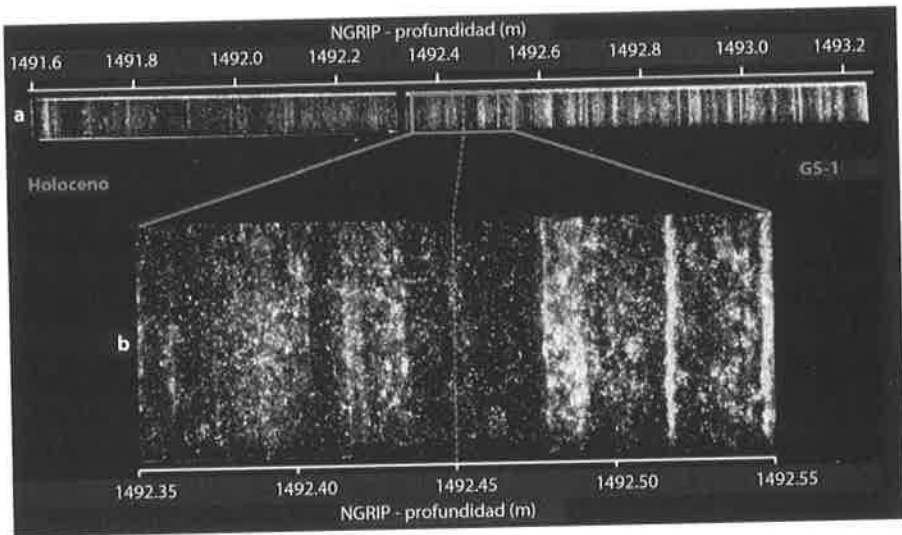
Figura 16.- Estratigrafía del sondeo de hielo NGRIP (Groenlandia). El bandeo anual en el hielo indica la señal estacional. El límite Pleistoceno-Holoceno se sitúa a 1492,45m de profundidad del sondeo (Walker et al., 2009).
