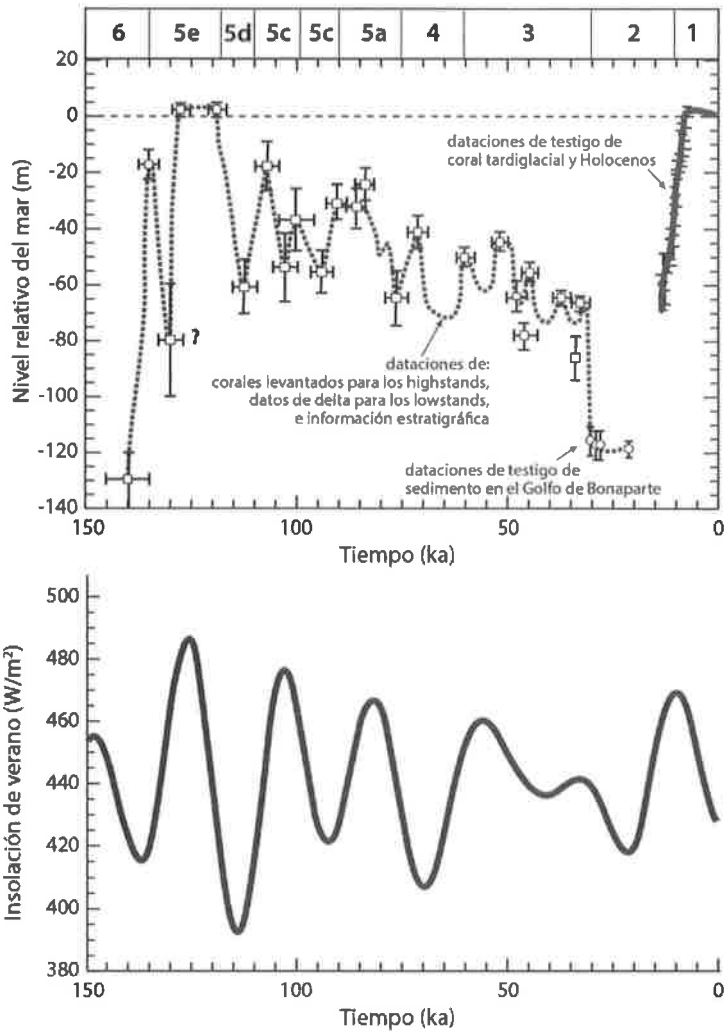
Figura 11.-Cambios del nivel del mar durante el último ciclo glacial, y comparación con la variabilidad de la insolación de verano (julio, 65° N). La curva del nivel del mar se ha elaborado a partir de los datos de la península de Huon (Nueva Guinea) y los del Golfo de Bonaparte (Australia). Según Lambeck et al. (2002). Obsérvese cómo, durante ese tiempo, las oscilaciones del nivel del mar son mucho más numerosas y rápidas que las de la insolación. No obstante, el nivel global más bajo del mar (entre 120 y 140 m bnm ) coincidió aproximadamente con el máximo volumen de hielo de los casquetes, hacia los 21 ka, es decir durante el MIS 2.
