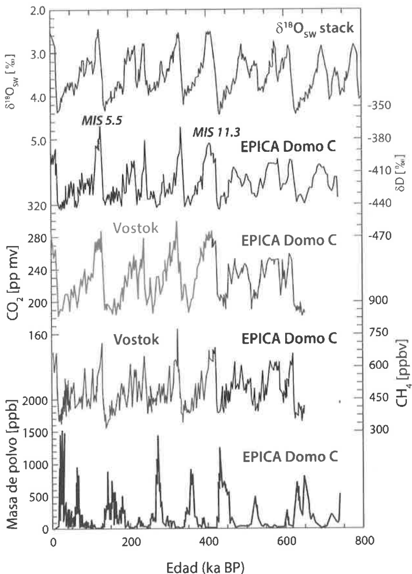
Figura 7.- Parámetros de los sondeos en la Antártida, Vostok y EPICA-Domo C, para los últimos 750 ka, comparándolos con los datos del \delta^{18}\text{O}\% de foraminíferos bentónicos en sondeos marinos (Lisiecki y Raymo, 2005). Se han señalado los óptimos o picos de los interglaciares MIS 5 (subpiso MIS 5.5) y MIS 11 (Subpiso MIS 11.3). Según Wolff (2006).
