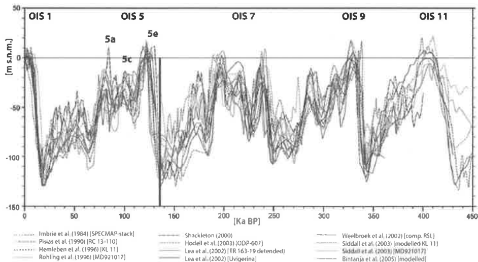
Figura 1.- Curvas seleccionadas del nivel del mar para los ciclos más recientes. Las curvas de líneas continuas representan el nivel relativo del mar (RSL), las discontinuas se corresponden con el nivel del mar derivado (Derived RSL). Interglaciares = OIS (Oxigen Isotope Stage): OIS 1- Presente Interglaciario, OIS 5 -Último Interglaciario, OIS 7 -Penúltimo Interglaciario, etc. (Según Caputo, 2007). 5a, 5c, 5e, highstands del OIS 5.
