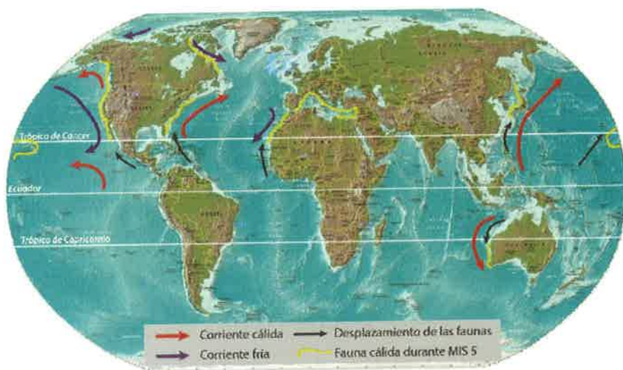
Figura 10.- Principales desplazamientos de moluscos marinos de aguas superficiales costeras desde los trópicos hasta las latitudes medias (flechas negras) y costas (en amarillo) con presencia de especies cálidas durante el MIS 5, hoy en día ausentes en esas zonas. Las flechas rojas indican las trayectorias de las aguas cálidas, las flechas azules las trayectorias de las corrientes frías (varios autores, sintetizado por Cabero et al. , 2013).
