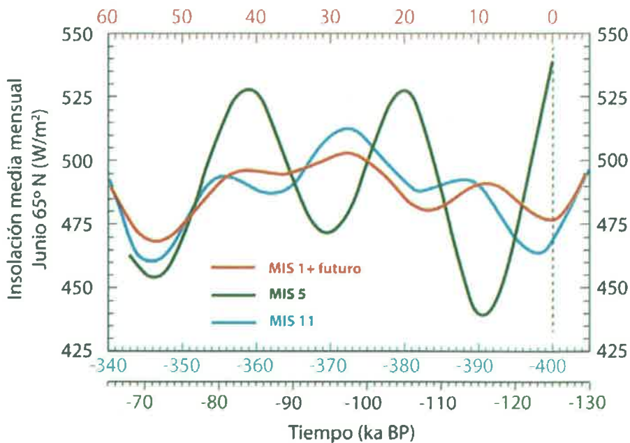
Figura 6.- Comparación entre las variaciones de la insolación de verano (mediados de Junio) a 65° N, durante los interglaciares correspondientes al MIS 11, último interglaciar MIS 5 y presente interglaciar MIS 1 (según Loutre y Berger, 2003).
