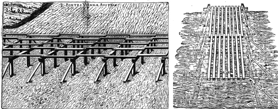
(3) Izqda.: Verancio, Pontes Viennae Austriae . (4) Dcha.: Puente flotante. Palladio 1650: 160
