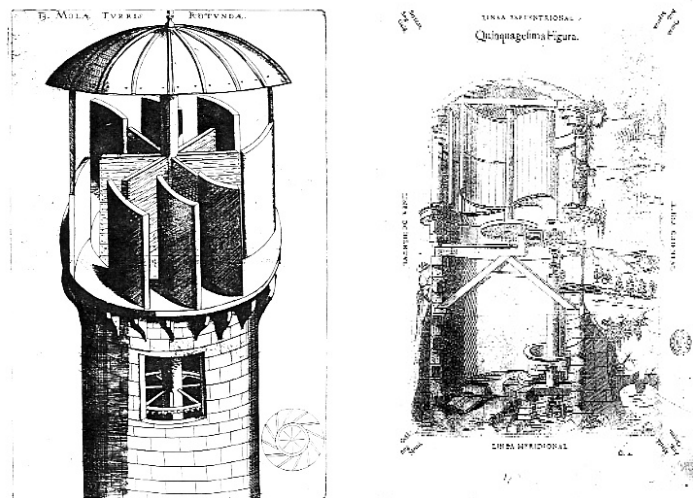
(1) Izqda.: Verancio, lámina 13: Mola Turris Rotunda ; (2) dcha.: Besson, Teatro de los instrumentos y figuras , 1602.
